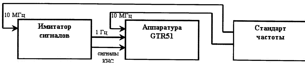
Рисунок 1 – Схема рабочего места для определения допустимого СКО случайной составляющей инструментальной погрешности измерений псевдодальности до навигационного космического аппарата
