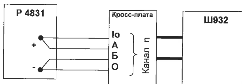
Рисунок Б.6 - Схема для проверки каналов сопротивления Ш932.7, Ш932.9 по 4-х проводной схеме
