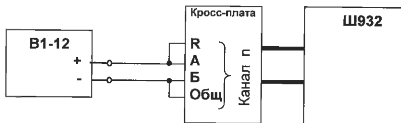
Рисунок Б.4 - Схема для проверки каналов тока Ш932.7, Ш932.9
