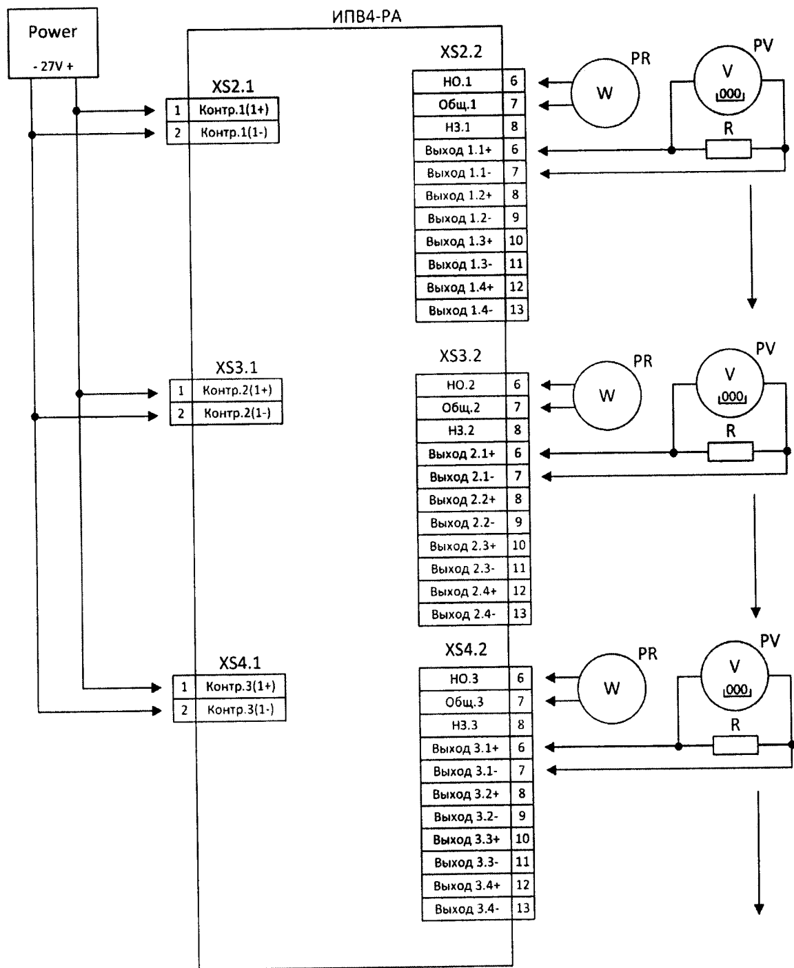
Рисунок А.2-Определение стабильности нуля расходомеров с электропитанием от сети переменного тока напряжением 220 В.
