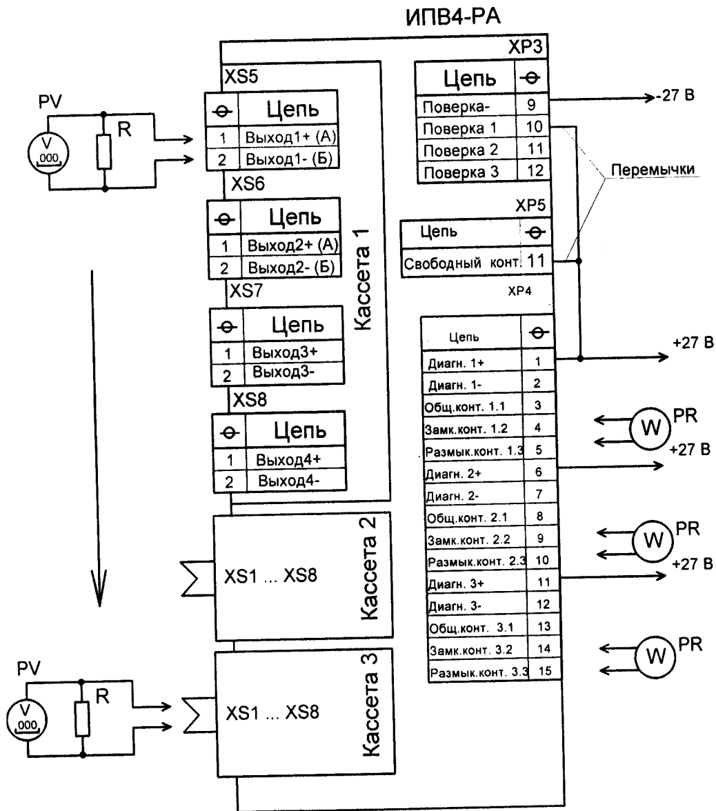
Рисунок А.1-Определение стабильности нуля расходомеров с электропитанием от сети постоянного тока напряжением 24 или 27 В. Остальное – см. схему соединений РИОУ.407254.002 РЭ
