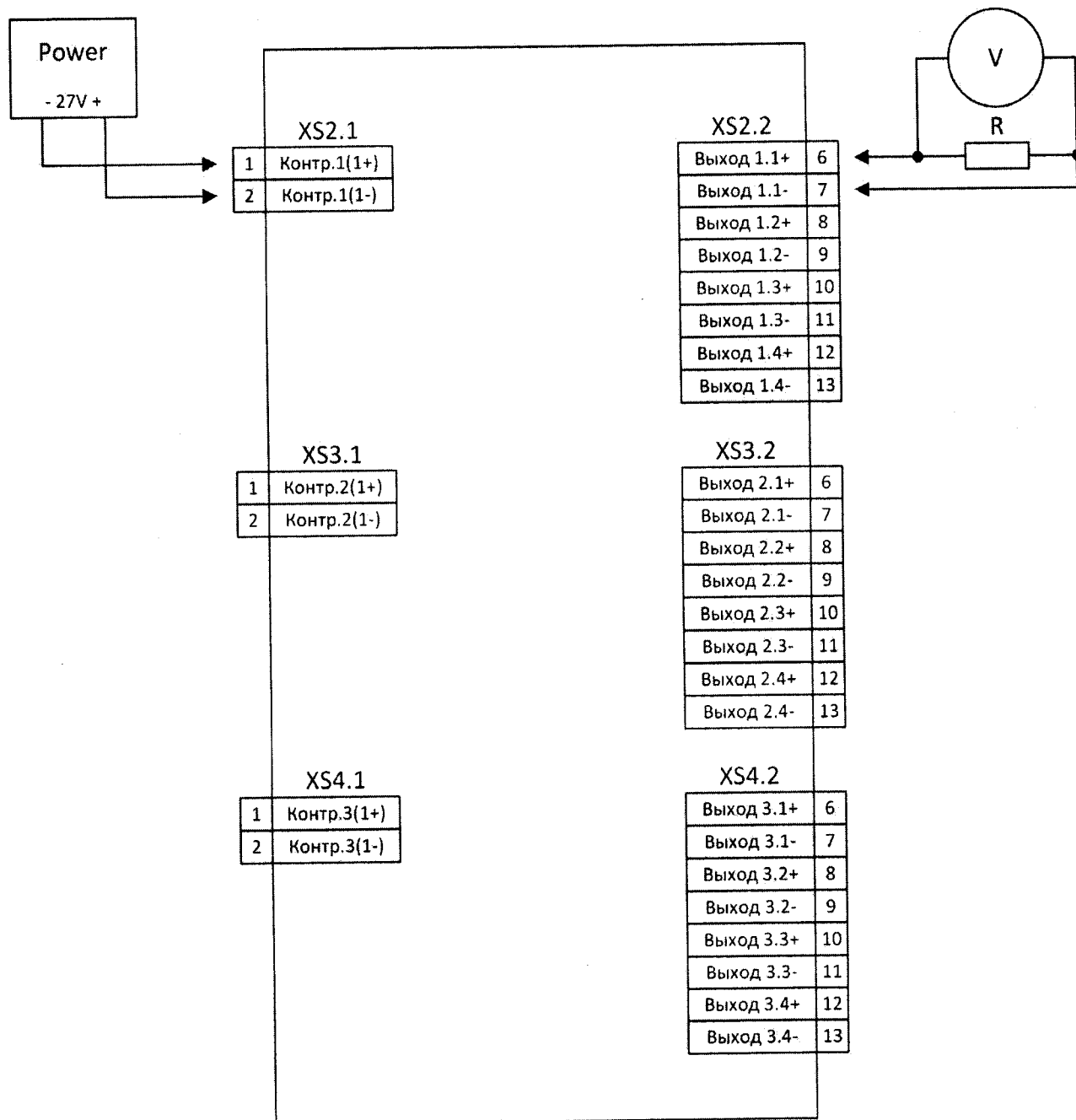
Рисунок А.6- Имитация точки расхода 0,9 Q_{\max} расходомеров с электропитанием от сети переменного тока напряжением 220 В. Остальное см. рисунок А.2
