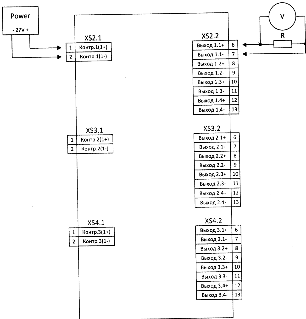
Рисунок А.4- Имитация точки расхода 0,5 Q_{\max} расходомеров с электропитанием от сети переменного тока напряжением 220 В. Остальное см. рисунок А.2
