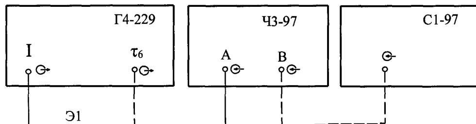
Рисунок 7.3 Схема соединения приборов при определении диапазона измерения длительности фронта/спада импульсов по входам А и В
