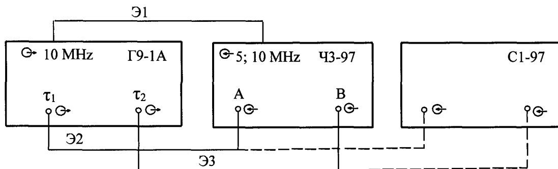
Рисунок 7.11 Схема соединения приборов при проверке аппаратурной разрешающей способности измерения интервалов времени.
