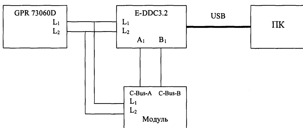
Рисунок 1 – Схема подключения модулей при опробовании и подтверждении соответствия программного обеспечения
