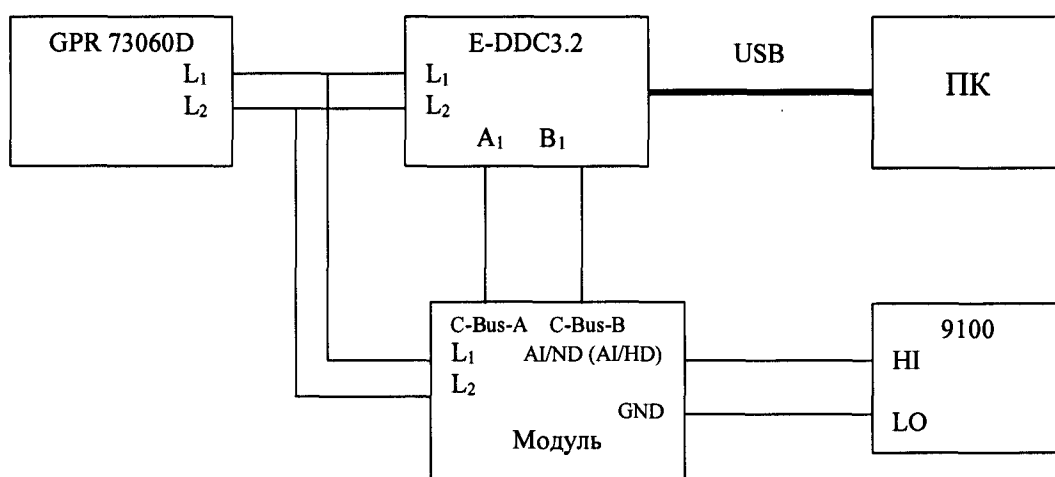
Рисунок 2 – Схема подключения модулей при определении относительной погрешности измерений напряжения постоянного тока
