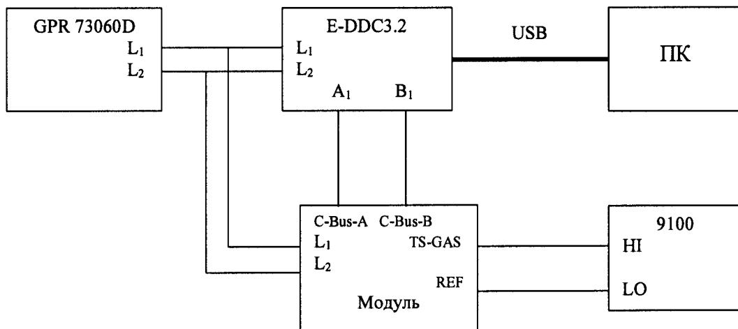
Рисунок 2 – Схема подключения модулей при определении абсолютной погрешности измерений сигналов от термопреобразователей сопротивления
