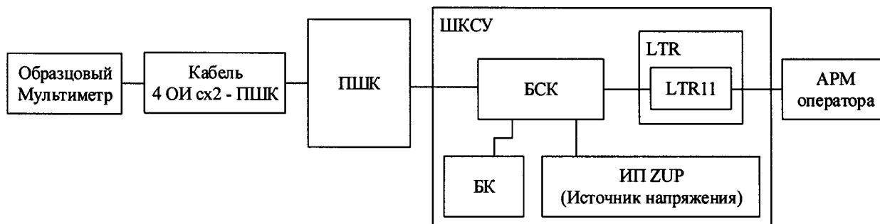
Рисунок 3 - Схема подключения вспомогательного оборудования и эталонных средств при проверке ИК напряжения постоянного тока
