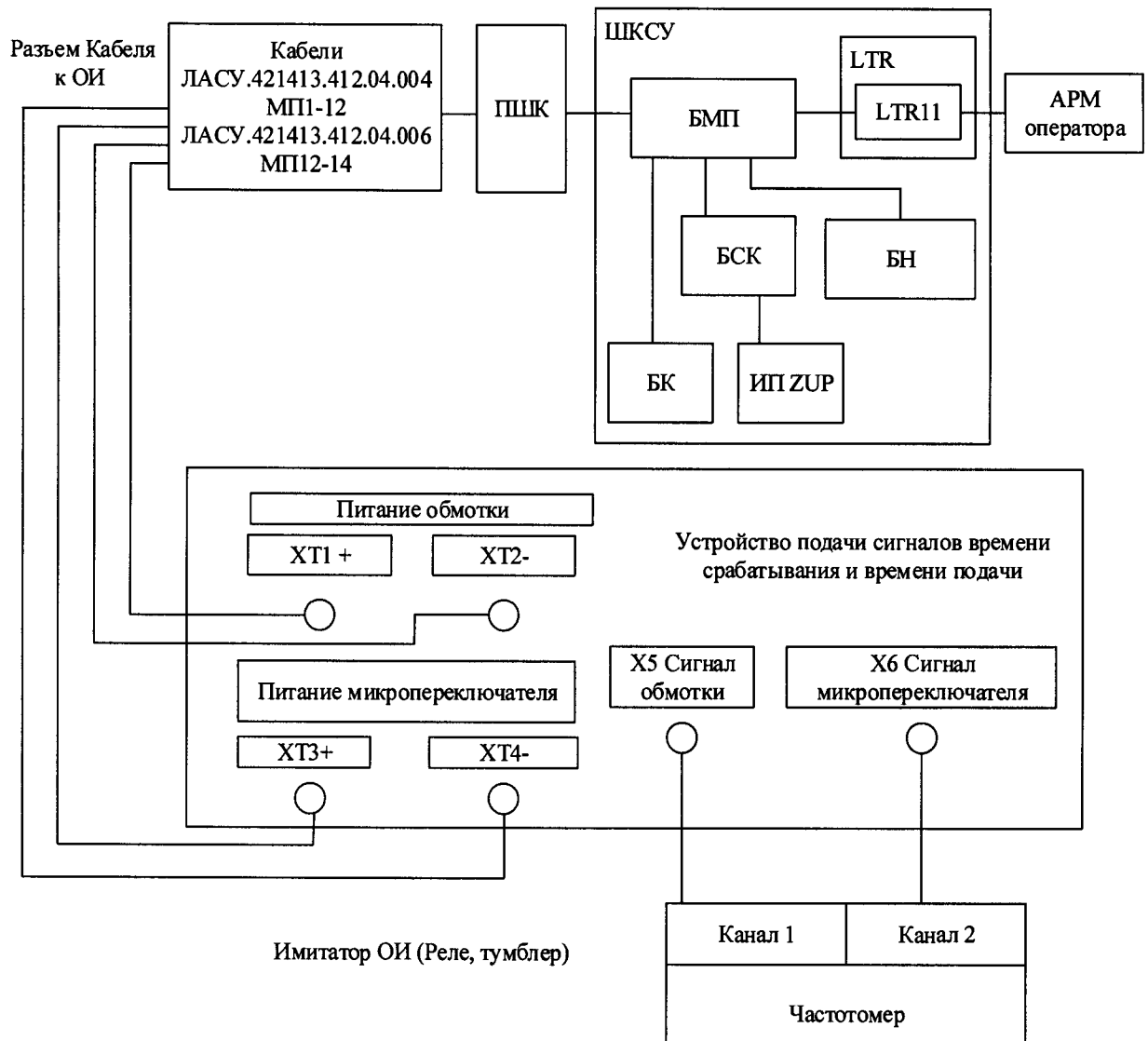
Рисунок 5 – Схема подключений вспомогательного оборудования и эталонных средств при проверке ИК временных интервалов.
