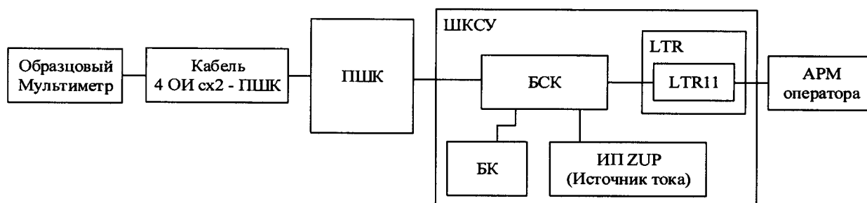
Рисунок 1 - Схема подключений вспомогательного оборудования и эталонных средств при поверке ИК силы постоянного тока.
