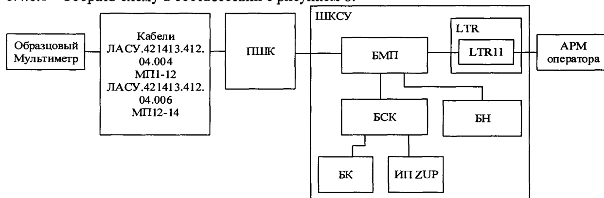
Рисунок 8 - Схема подключений вспомогательного оборудования и эталонных средств при поверке ИК воспроизведения силы постоянного тока
