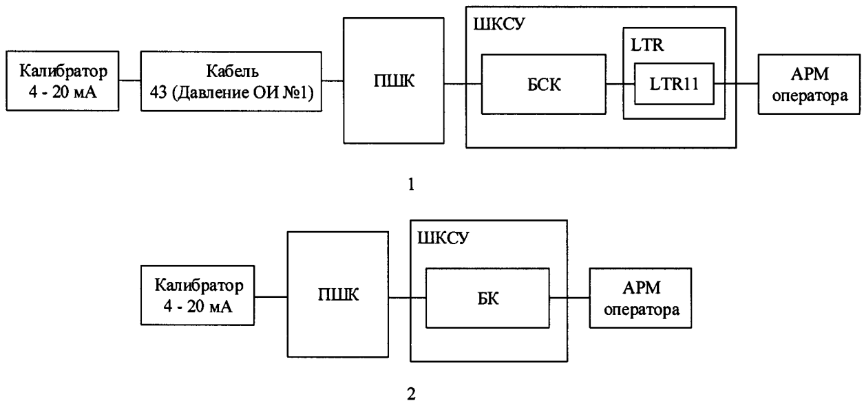
Рисунок 4 Схема подключений вспомогательного оборудования и эталонных средств при проверке ИК избыточного давления.
