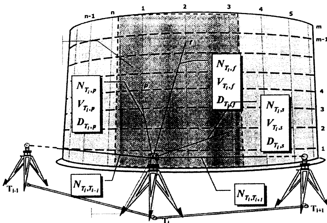
Рисунок А.4 – Измерения тахеометром при определении горизонтальных координат и абсолютной высоты точек на поверхности резервуара
