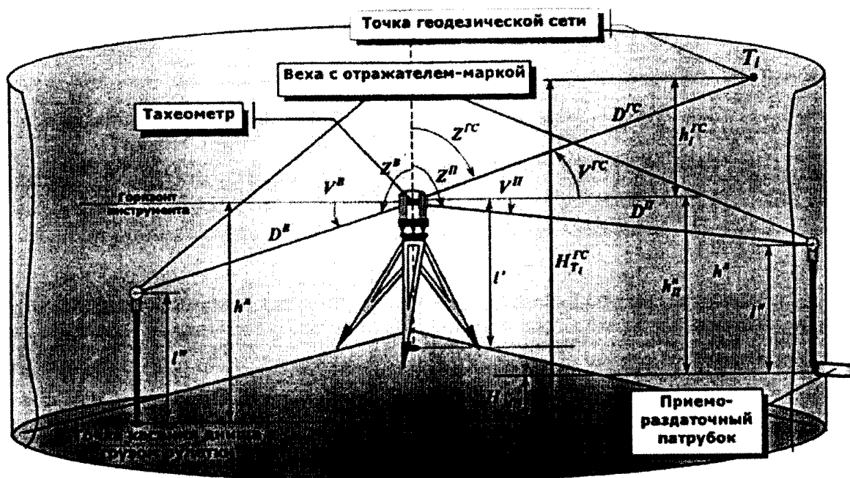
Рисунок А.3 Определение абсолютной высоты точки геодезической сети и „мертвой” полости относительно точки касания дна грузом рулетки при установке тахеометра внутри резервуара
