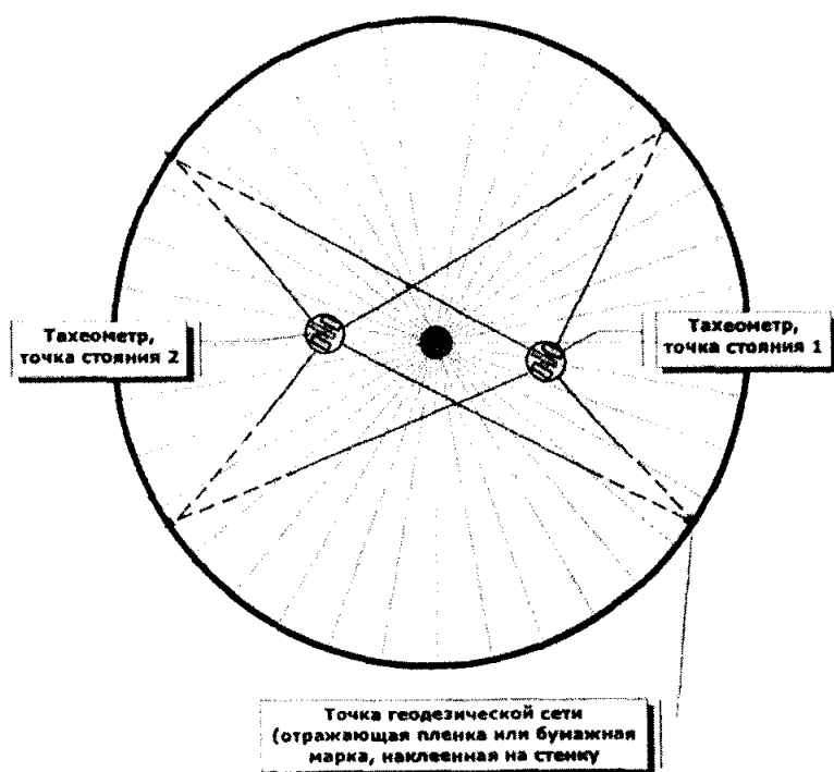
Рисунок А.2 Схема геодезической сети при выполнении измерений внутри резервуара
