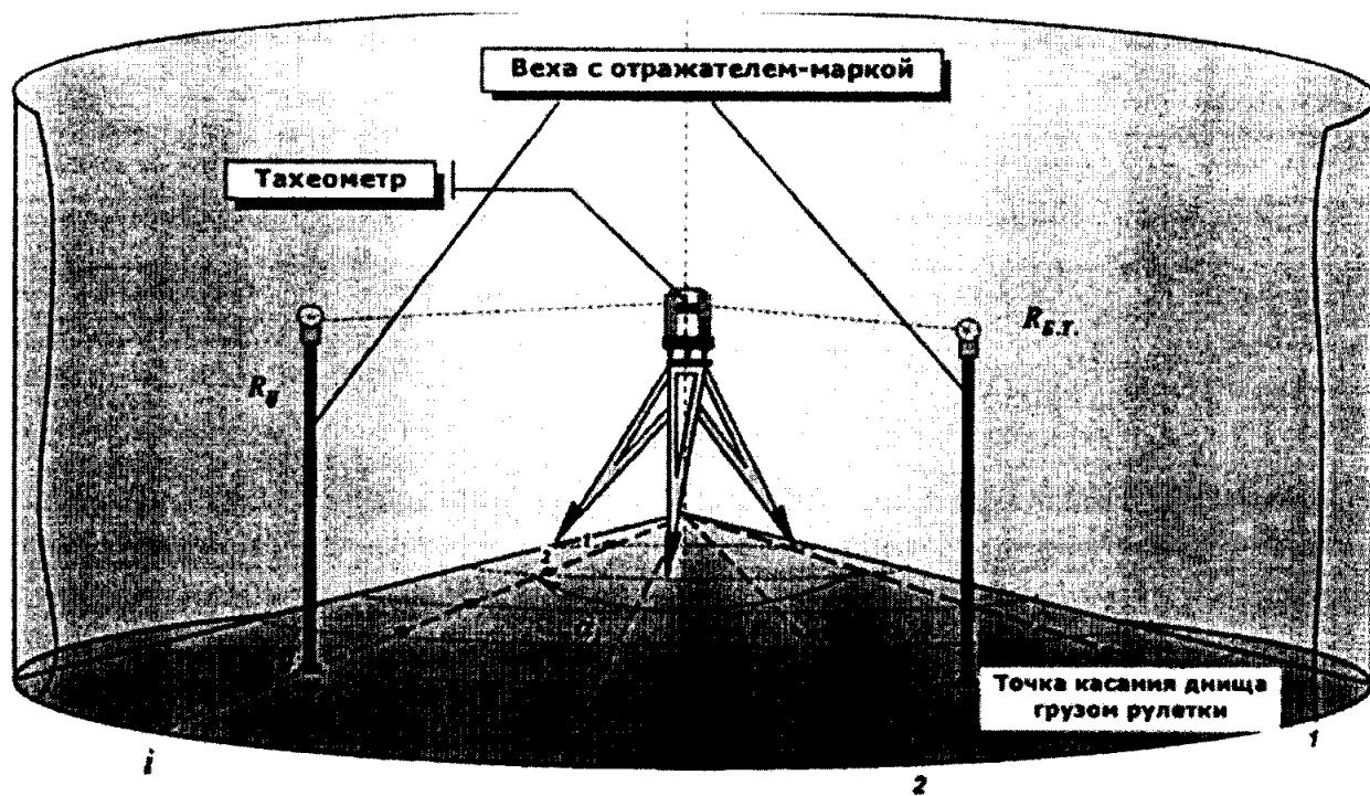
Рисунок А.6 Определение параметров дна резервуара
