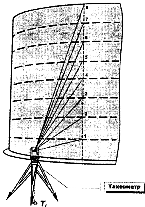
Рисунок А.5 Определение абсолютной высоты поясов тригонометрическим нивелированием
