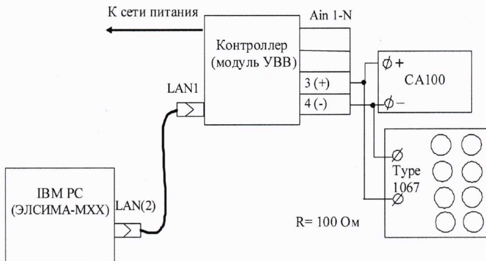
Рисунок 2 – Схема проверки погрешности измерения силы постоянного тока для контроллера Элсима-MXX и модуля Элсима-DAXX
