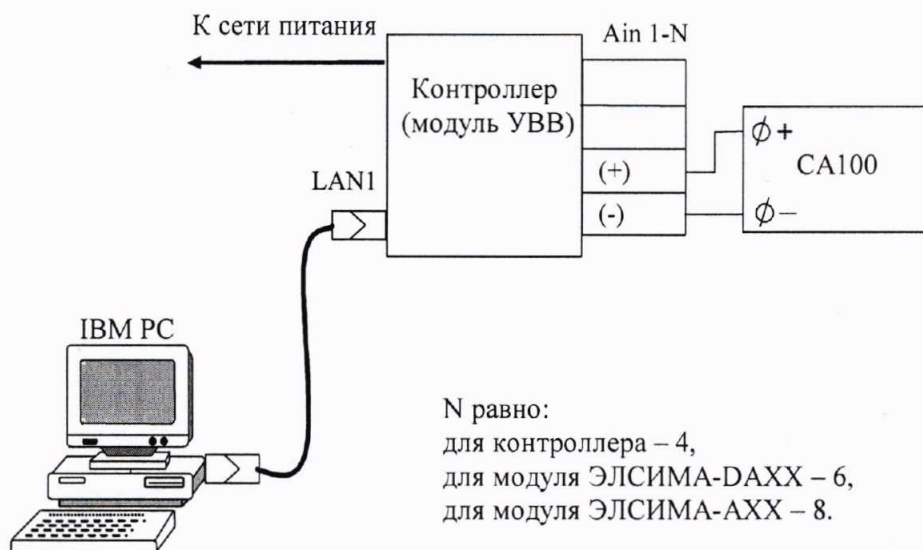
Рисунок 6 – Схема проверки погрешности преобразования сигналов термопреобразователей напряжения (термопар)
