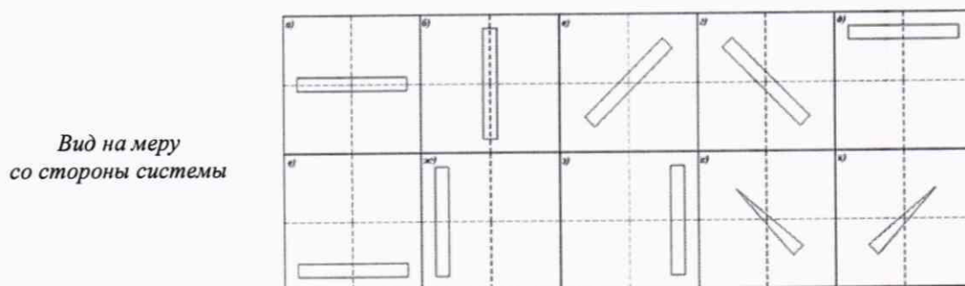
Рисунок 2 – Мера расположена под углом 0° (а), 90° (б), +45° (в), -45° (г), +Y (д), -Y (е), -X (ж), +X (з), объемная диагональ под углом -45° (и) и объемная диагональ под углом +45° (к)
