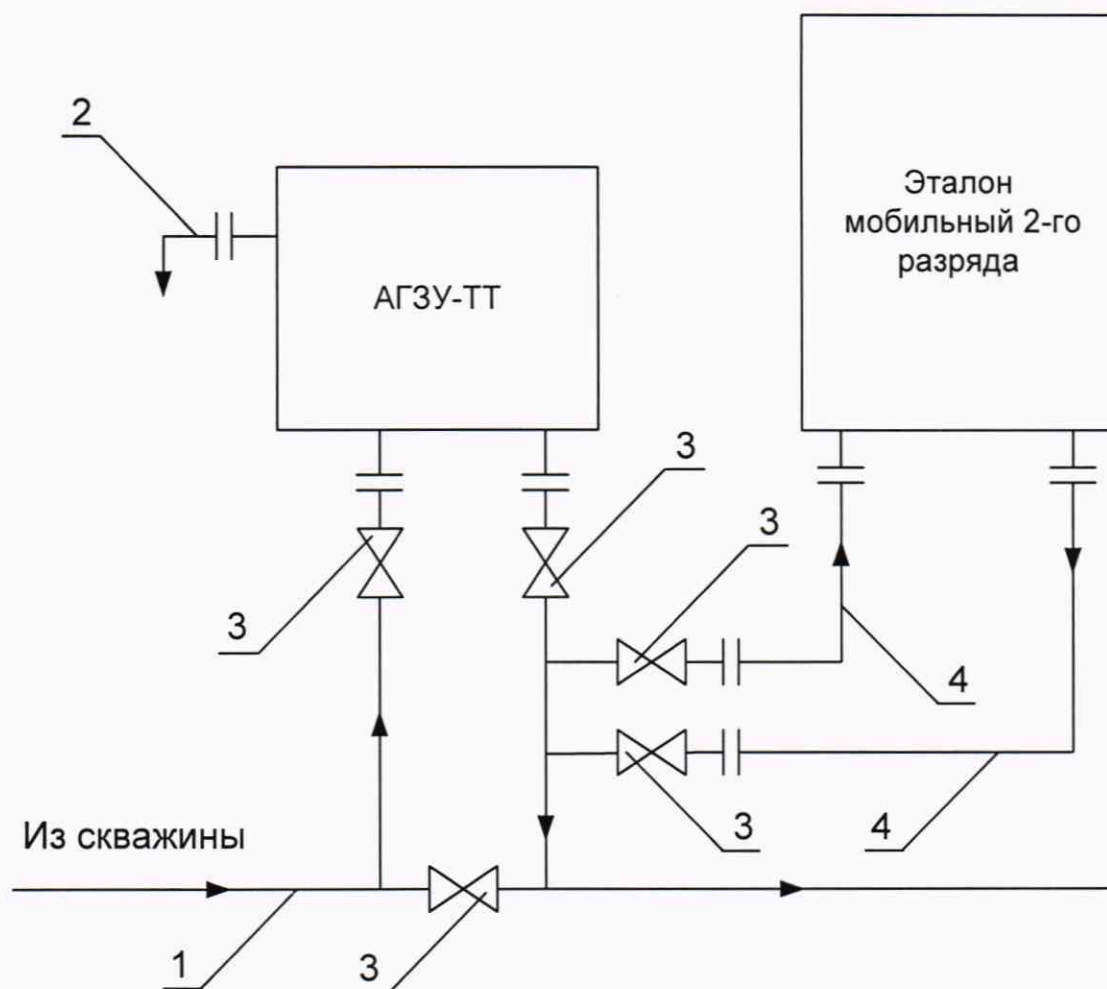
Рисунок А2. Гидравлическая схема подключения установки при поверке на месте эксплуатации
