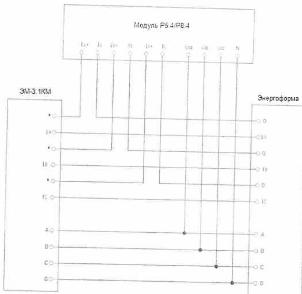
Рисунок 9 – Схема подключений терминала для проверки модуля Р5.4/Р8.4 (с опцией РМ)
