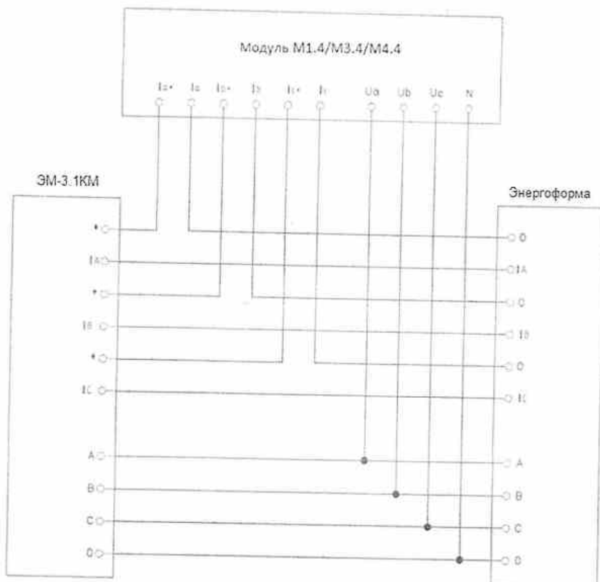
Рисунок 8 – Схема подключений терминала для проверки модуля M1.4/M3.4/M4.4 (с опциями M, QA)
