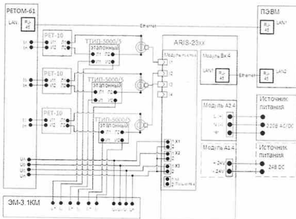
Рисунок 6 – Схема подключений терминала для проверки модулей P5.4, P8.4
