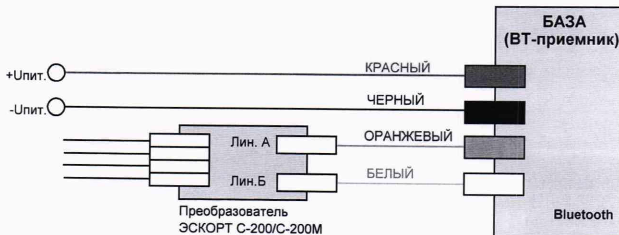
Рисунок А.1 – Схема подключения к ПК
