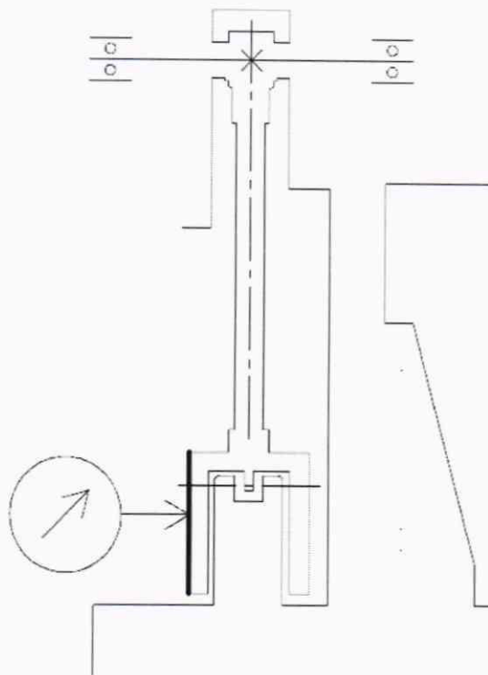
Рисунок 2– Установка индикатора для контроля отклонения \rho_l
