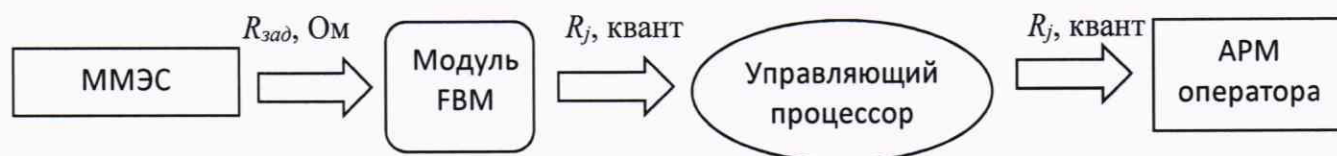
Рис. 1 - Схема подключения ММЭС и преобразования электрического сопротивления в цифровое значение
