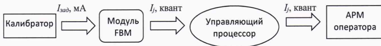
Рис. 2 - Схема подключения калибратора и преобразования токового сигнала в цифровое значение
