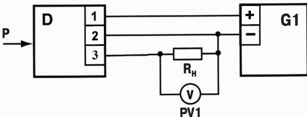
Рисунок Б.1 – Схема подключений преобразователей с выходным нормированным сигналом силы постоянного тока и цифровым интерфейсом HART
