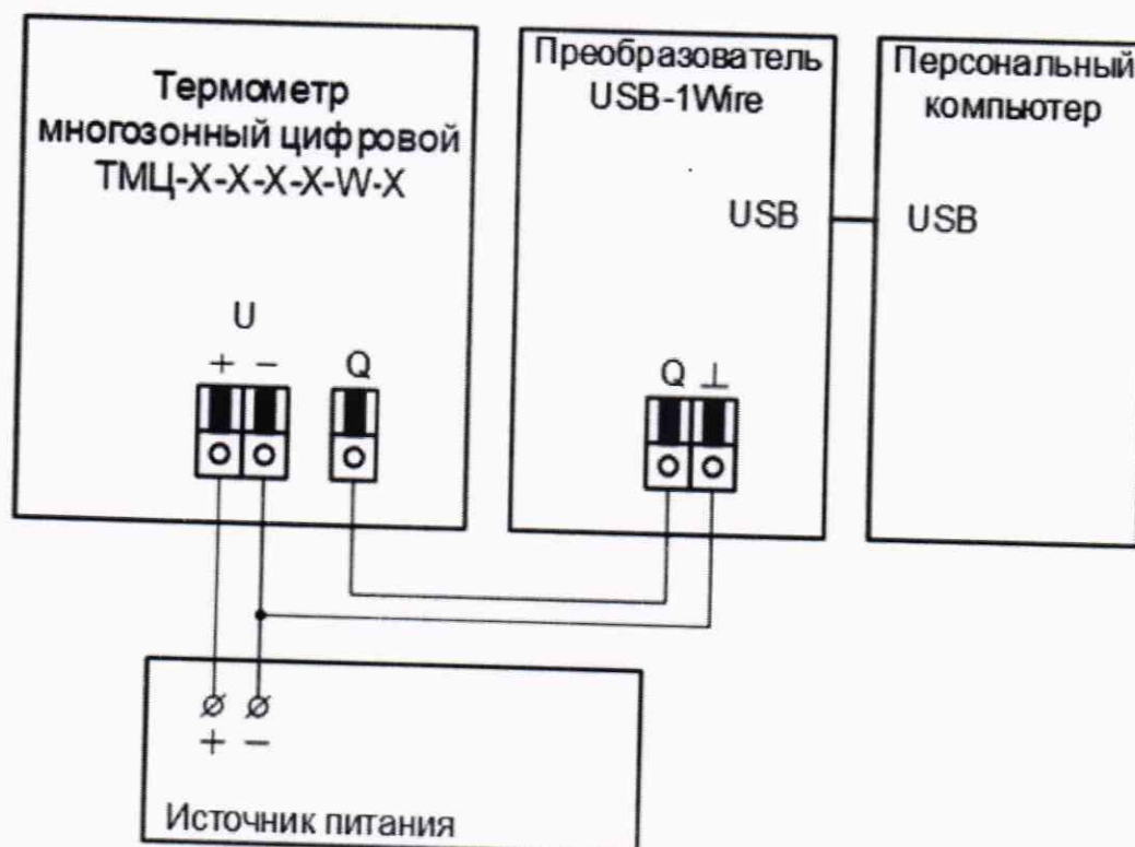
Рисунок А.2 – Схема соединений для проверки абсолютной погрешности измерений температуры и передачи измеренных значений по интерфейсу для модификации ТМЦ-X-X-X-X-W-X
