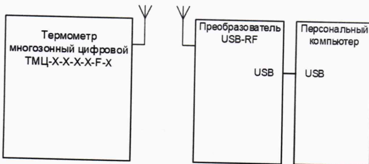
Рисунок А.4 – Схема соединений для проверки абсолютной погрешности измерений температуры и передачи измеренных значений по интерфейсу для модификации ТМЦ-X-X-X-X-F-X
