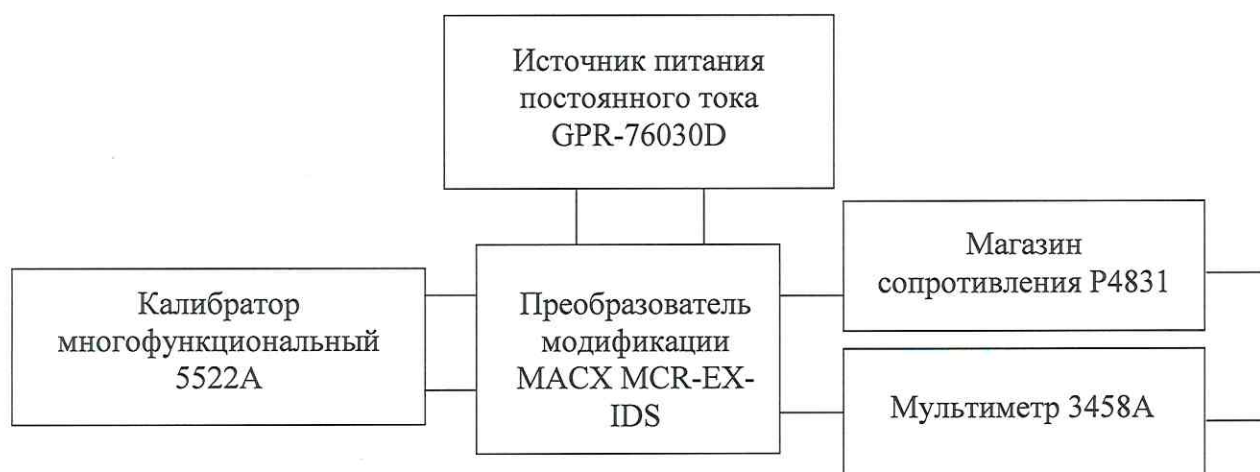
Рисунок 1 – Схема подключений для поверки преобразователя модификации MACX MCR-EX-IDS
