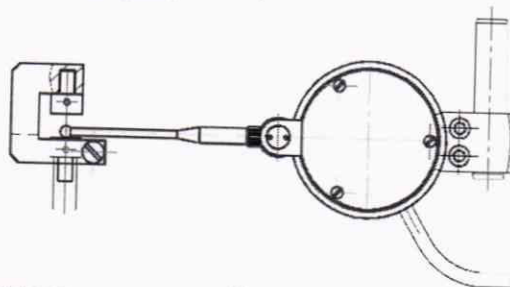
Рисунок 1 - Схема расположения преобразователей модели М-025 на приборе ППГ-4
