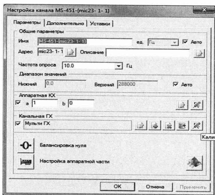
Рисунок 10 – Вид диалогового окна «Настройка канала...»
