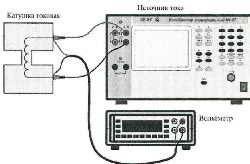
Рисунок 13.16 – Схема измерения сопротивления катушки токовой
