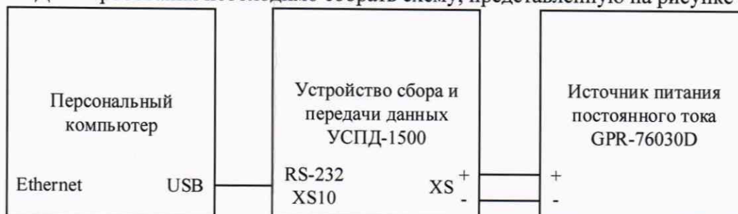
Рисунок 1 – Схема опробования
