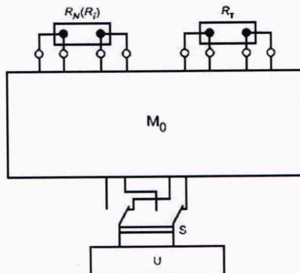
Рисунок А.1 - Подключение сравниваемых мер при использовании метода замещения
