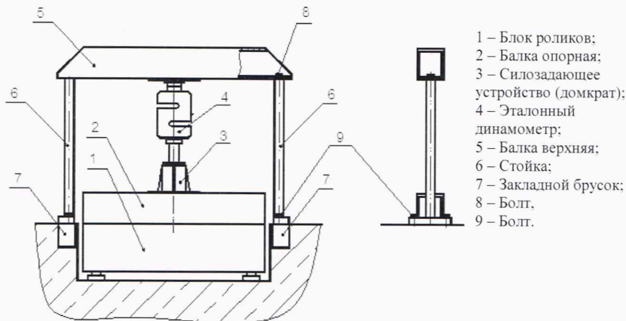
Рисунок 4 - Схема испытаний при определении относительной погрешности измерений массы транспортного средства, приходящейся на ось, для стенов модификаций мод. 1500-Z, мод. 3000М.01-Z, мод. 3000М.02-Z, мод. 3500-4, мод. 3500М-Z, мод. 6000-4/2, мод. 10000-Z, мод. 13000.01-Z, мод. 13000.02-Z, мод. 16000.01-Z
