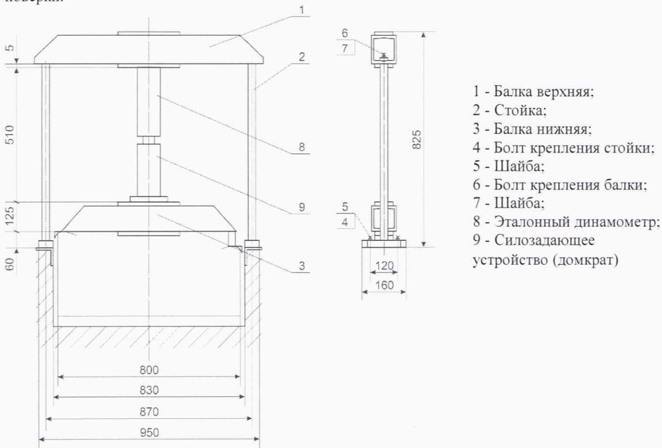
Рисунок 5 - Схема поверки при определении относительной погрешности измерений массы транспортного средства, приходящейся на ось, для стандов модификаций 16000.02-Z, 18000-4/2
