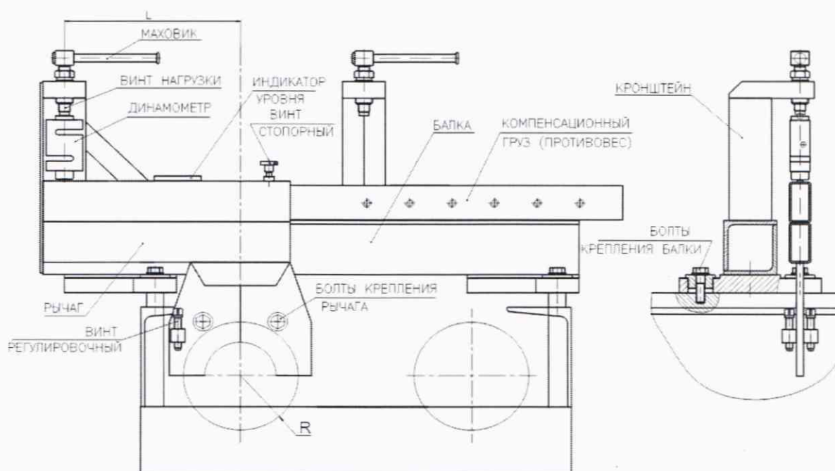
Рисунок А.1 - Рычаг поворочный для поверки датчиков тормозной силы стендов мод. 3000М.01-Z; мод. 3000М.02-Z, мод. 1500-Z, мод. 3500-4, мод. 3500М-Z, мод. 6000-4/2, мод. 10000-Z, мод. 13000.01-Z, мод. 13000-.02-Z, мод. 16000.01-Z
