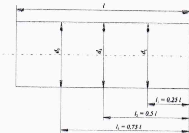
Рисунок 1 - Точки измерений для d_1 , d_2 и d_3
