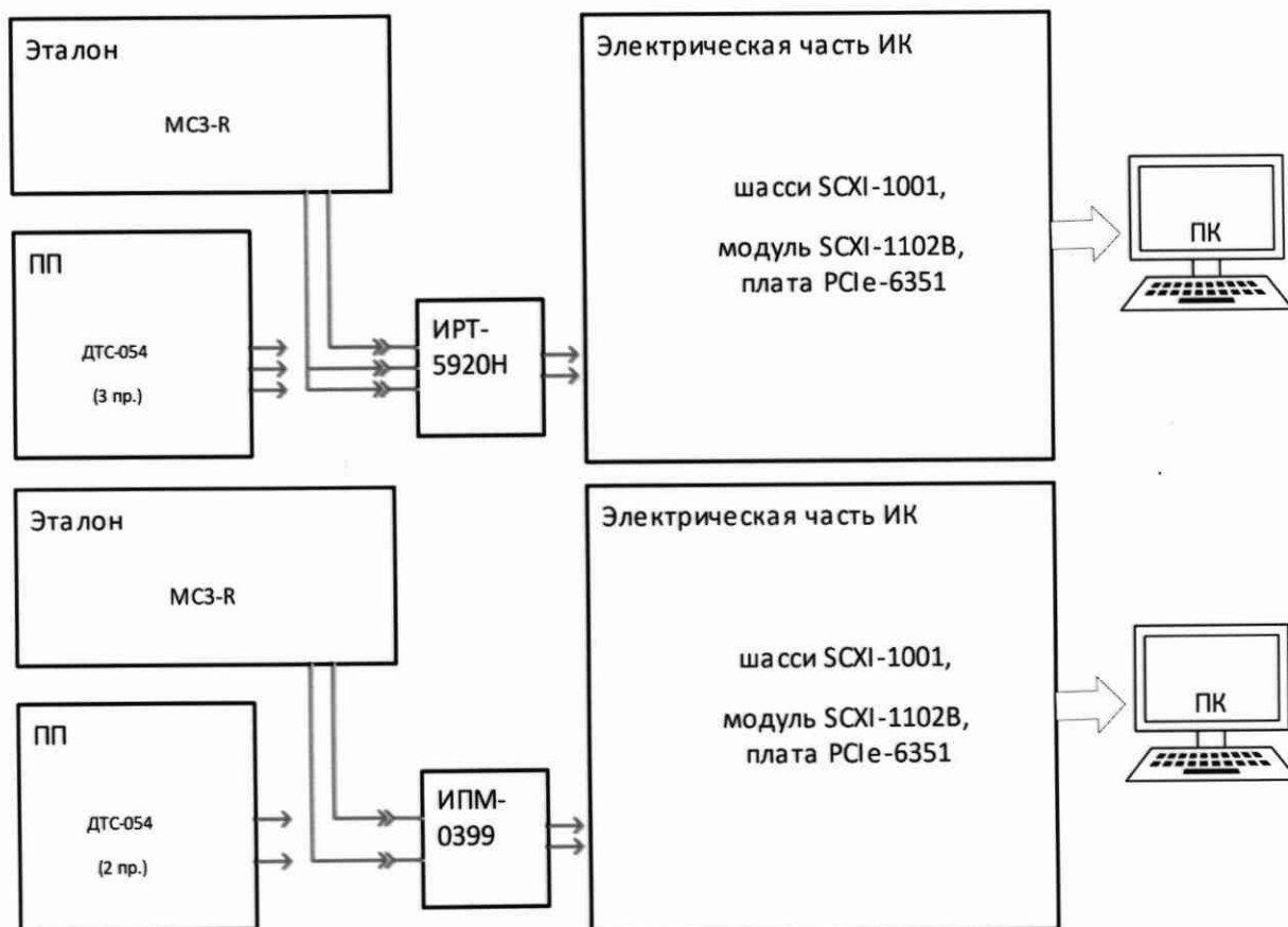
Рисунок 3 – Схемы поверки ИК температур газобразных и жидких сред поэлементным способом
