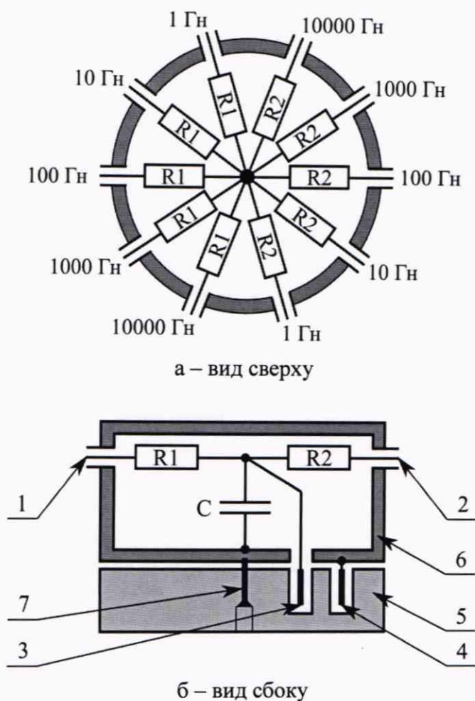
Рисунок 1 – Контактные выводы и размещение компонентов меры LQ-2408-3:
