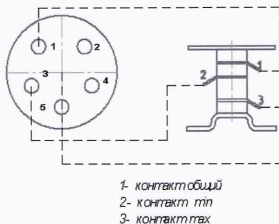
Рис.1-Схема внешних электрических соединений
