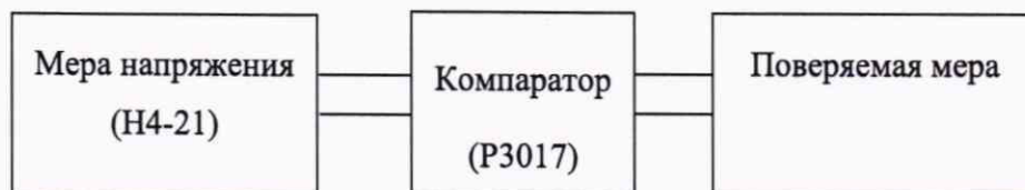
Рисунок 1 – Схема сличения поверяемой меры с эталонным СИ
