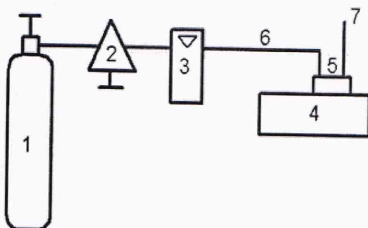
Рисунок Д.1.1 Схема определения относительной погрешности и времени срабатывания
