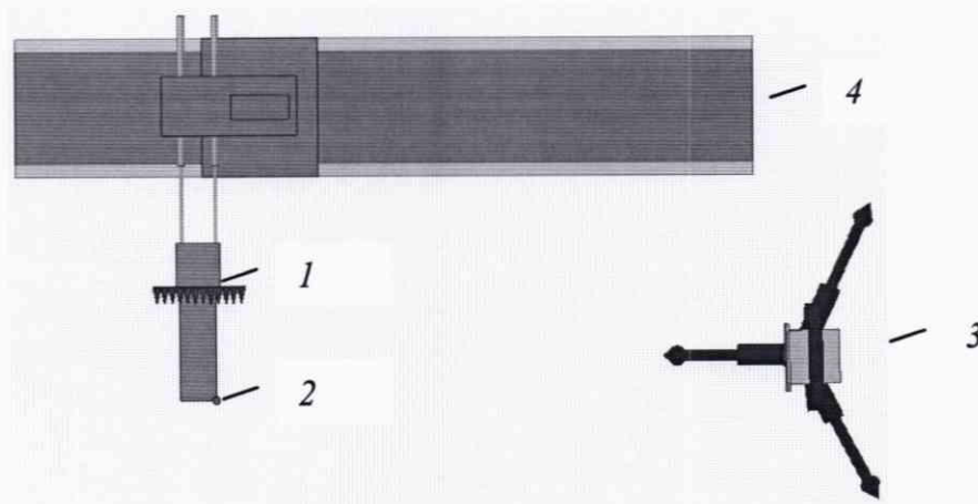
1 – антенна-зонд; 2 – оптический отражатель; 3 – система Leica AT401; 4 – сканер
