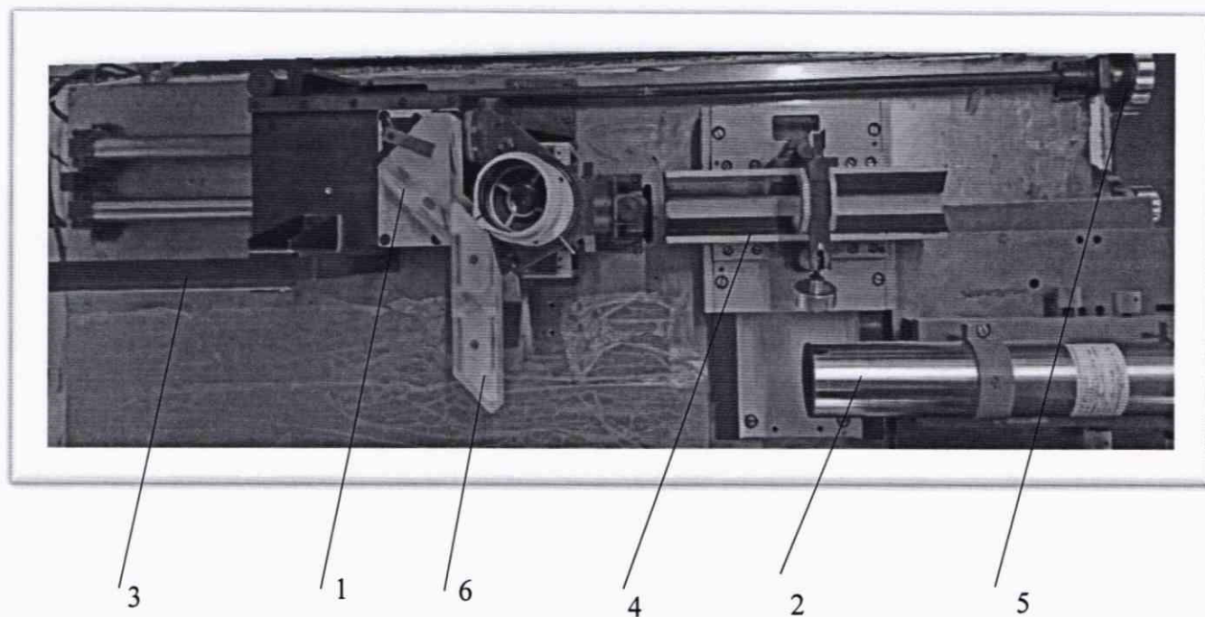
1 - призма ВкР-180°, 2 – автоколлиматор, 3 – шкала расстояний, 4 – посадочное место для труб визирных, 5 – рукоятка установки расстояний, 6 - ромб зеркальный.
