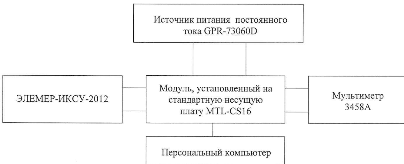
Рисунок 1— Схема подключений для поверки модуля в режиме аналогового ввода «АІ»
