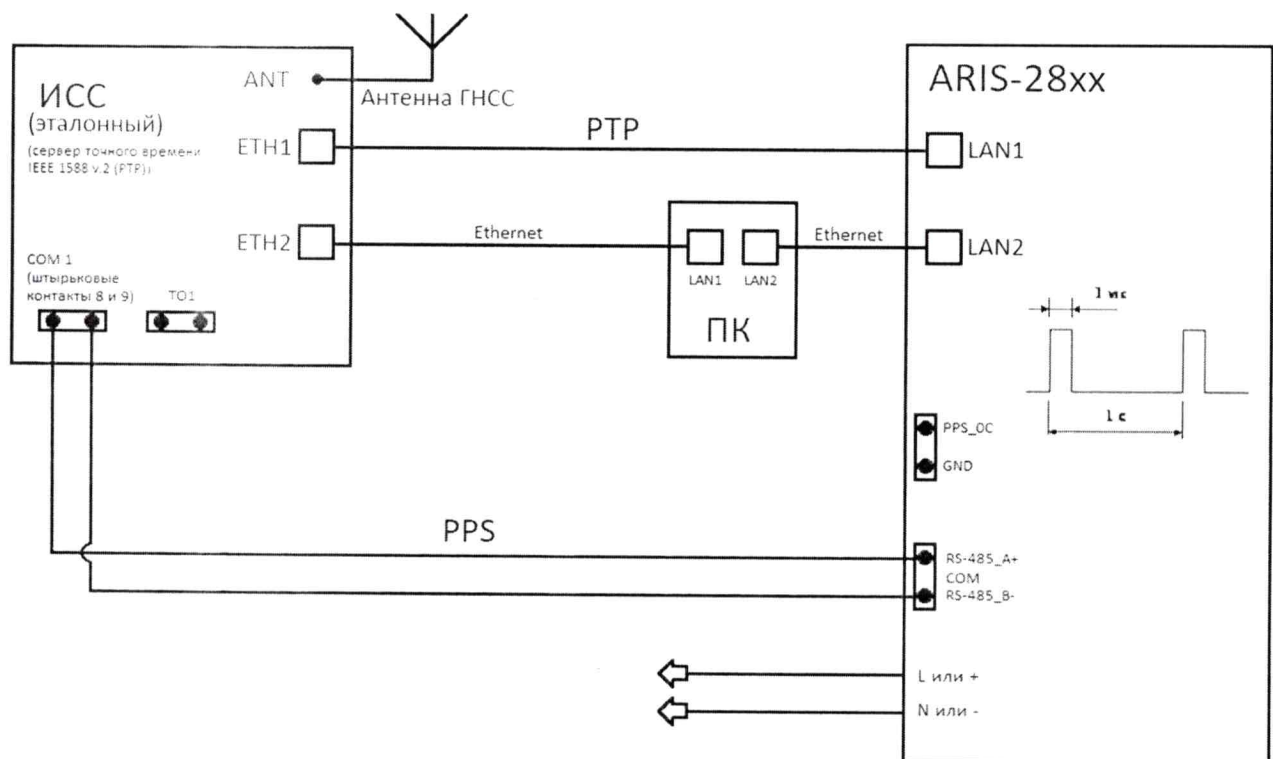
Рисунок 7 – Схема подключения при синхронизации от PTP-сервера
