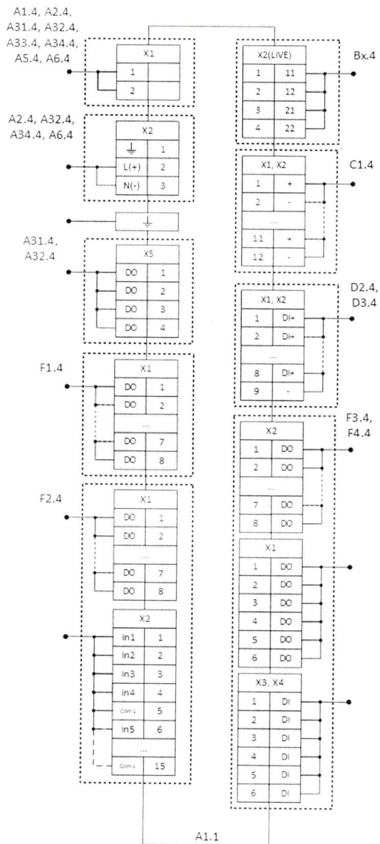
Рисунок 1 – Схема соединений для проверки электрической прочности изоляции цепей контроллера с номинальным напряжением свыше 60 В
