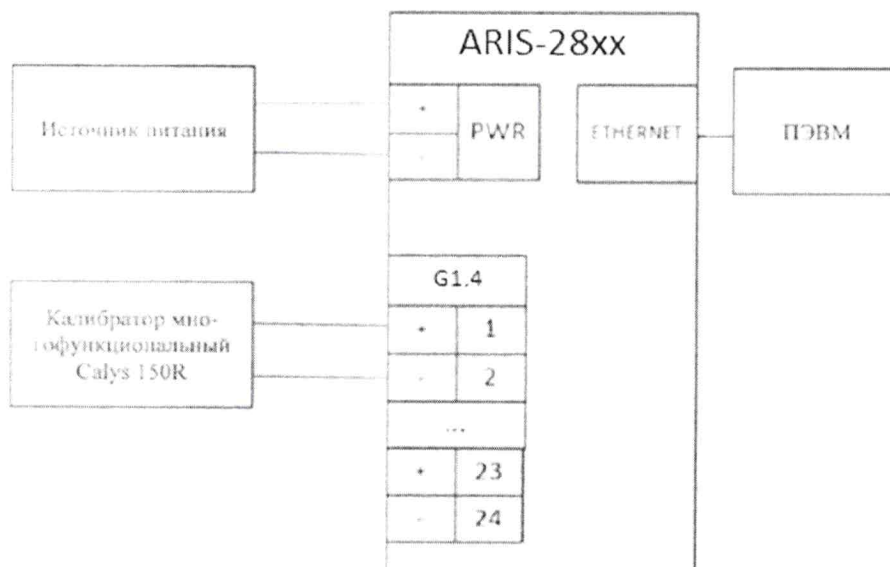
Рисунок 4 – Схема подключения при определении приведенной основной погрешности при измерении унифицированных аналоговых сигналов силы постоянного тока для модуля G1.4
