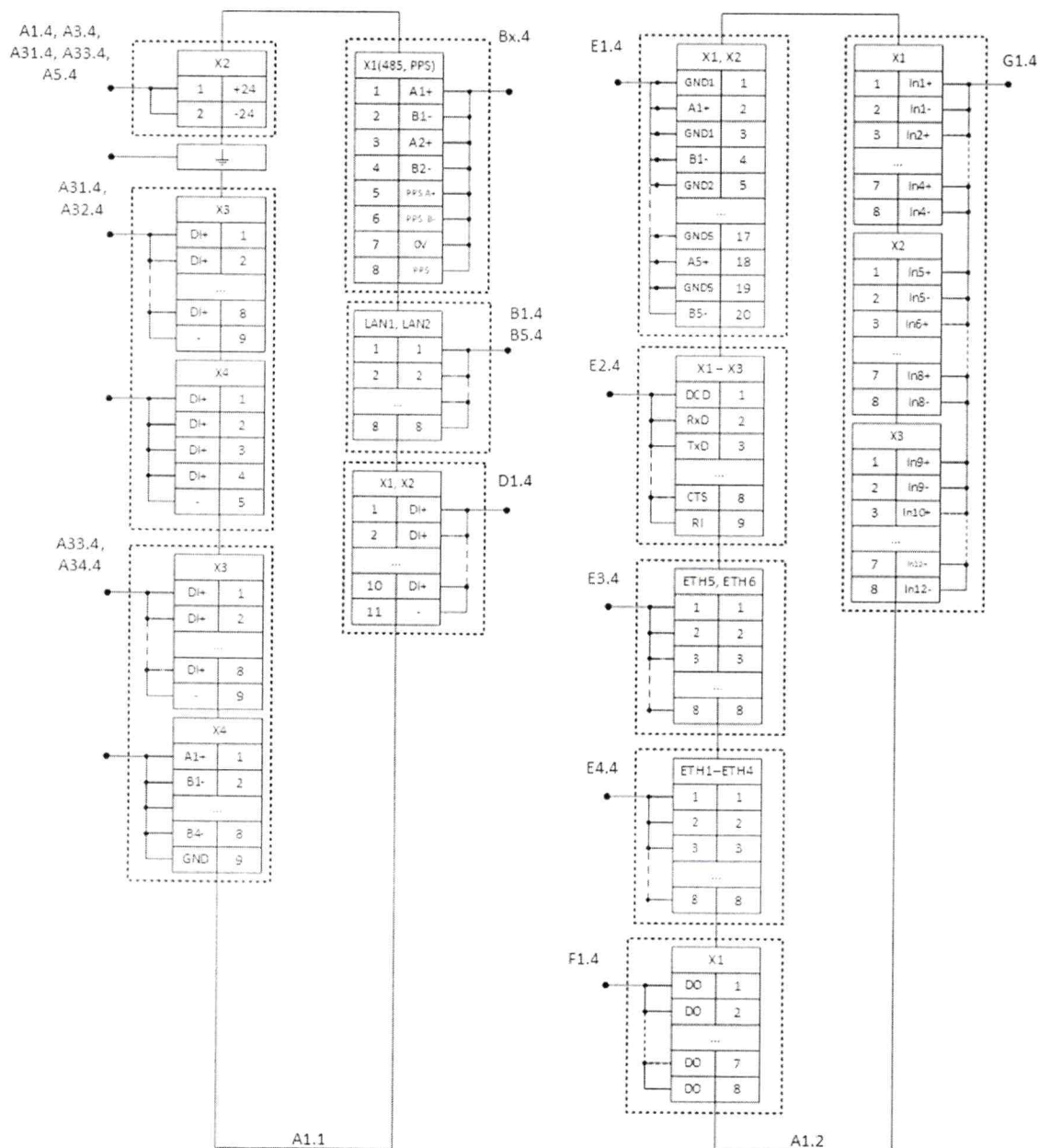
Рисунок 2 – Схема соединений для проверки электрической прочности изоляции цепей контроллера с номинальным напряжением не более 60 В
