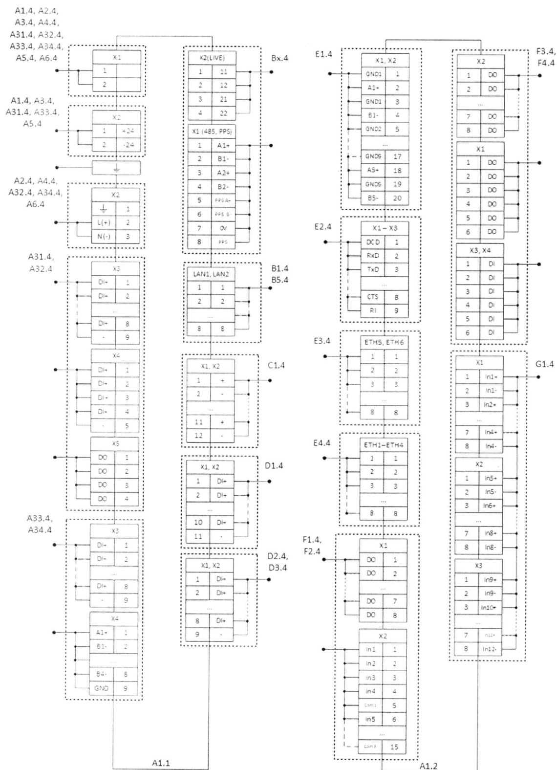
Рисунок 3 – Схема соединений для проверки сопротивления изоляции контроллера
