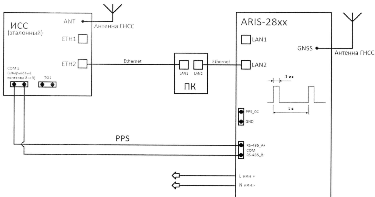
Рисунок 5 – Схема подключения при синхронизации от встроенного приёмника ГНСС
