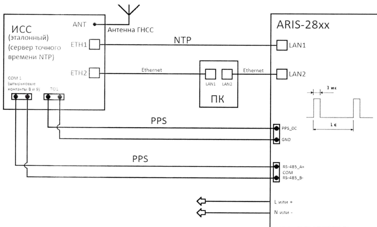
Рисунок 6 – Схема подключения при синхронизации от NTP-сервера
