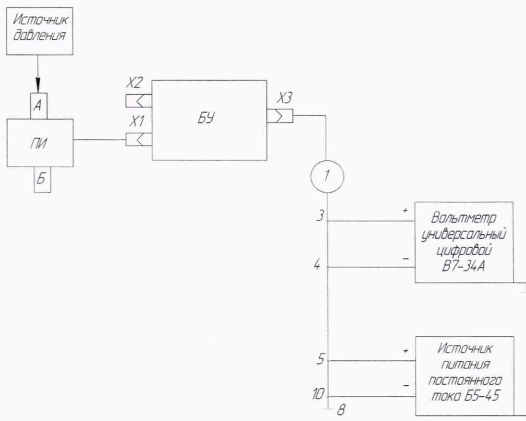
1 – кабель технологический Вм 6999-4249 Рисунок 1 – Схема для проведения испытаний
