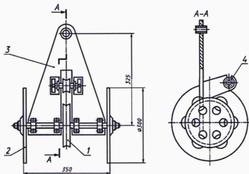
Рисунок А.3 - Измерительная каретка
