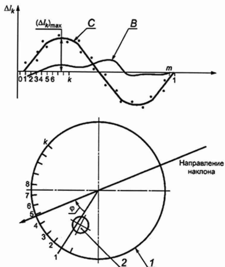
1 - контур днища резервуара; 2 - измерительный люк; \Delta I_k - функция, вычисляемая по формулам (4) и (5); С, В - графики функции \Delta I_k при наличии и отсутствии наклона резервуара соответственно; (\Delta I_k)_{\max} - максимум функции \Delta I_k ; m - число разбивок; k - номер разбивки; \varphi - угол направления наклона резервуара
