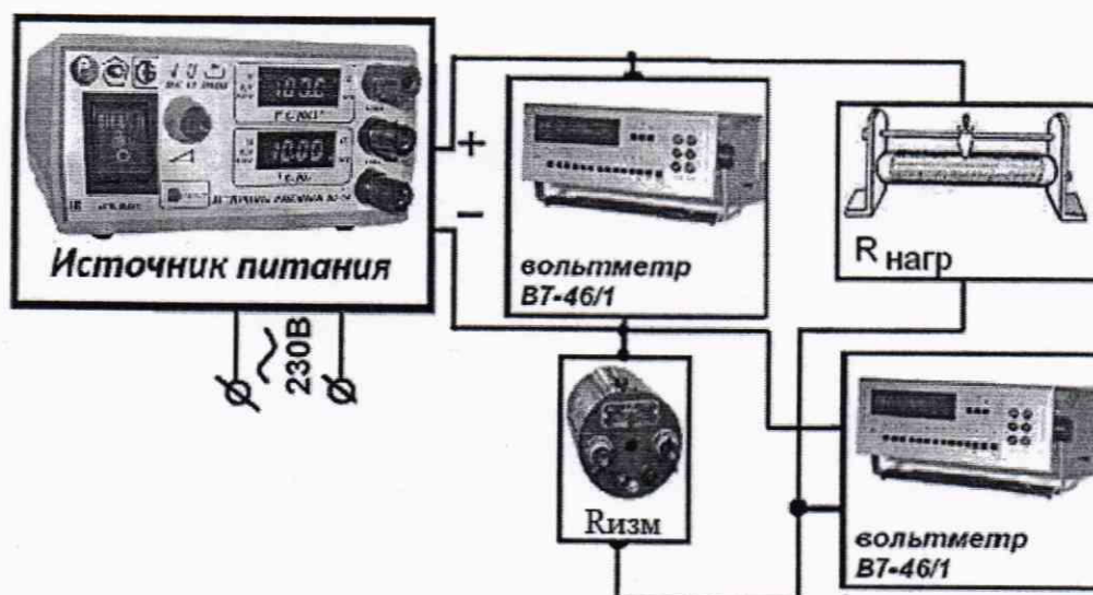
Рисунок 3 – Схема измерений нестабильности выходного напряжения ИП при изменении тока нагрузки и нестабильности выходного тока ИП при изменении напряжения на нагрузке
