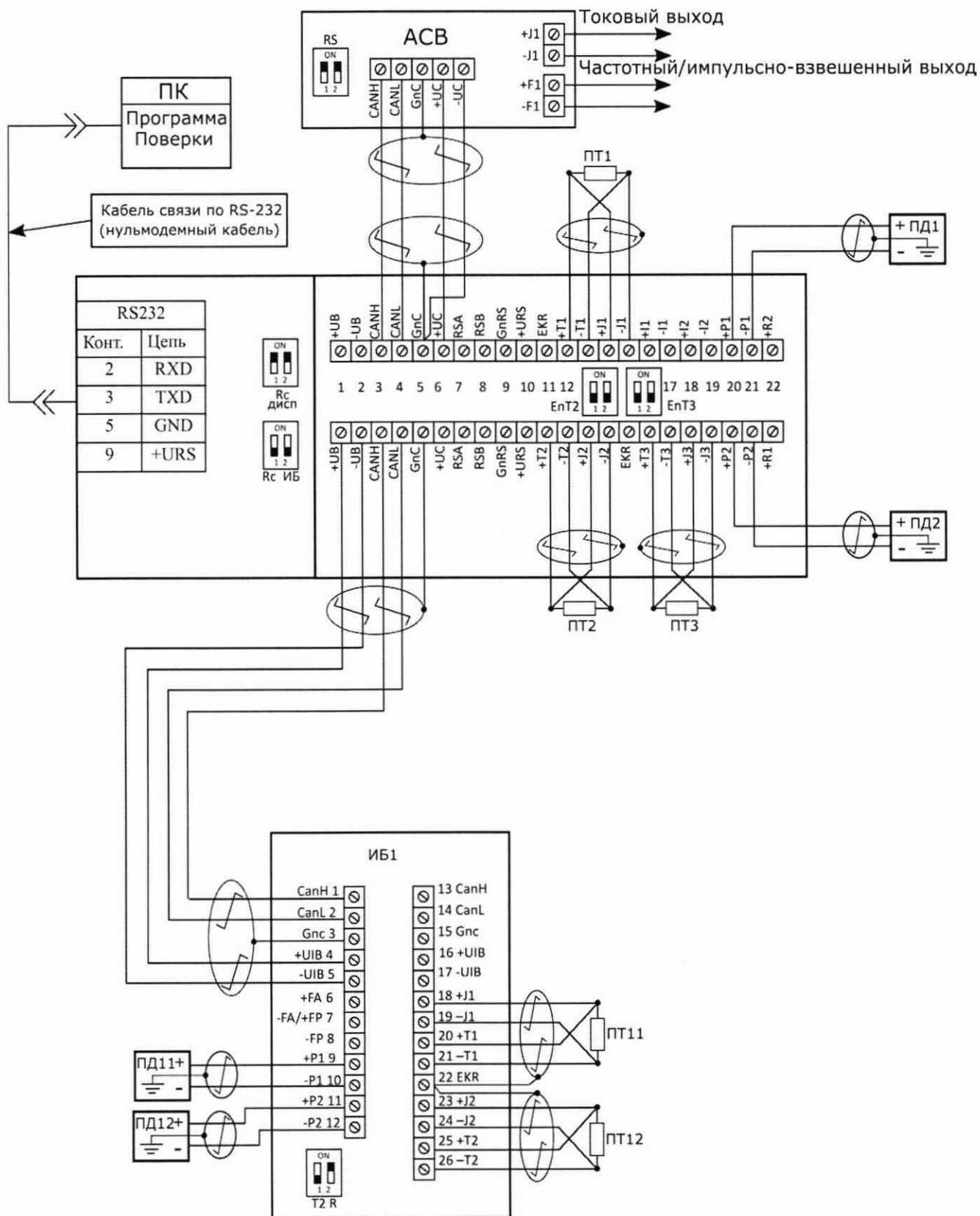
Рисунок А.3 – Электрическая схема подключения однопоточного теплосчётчика с ТеРосс-ИБ, имеющего цифровой выход
