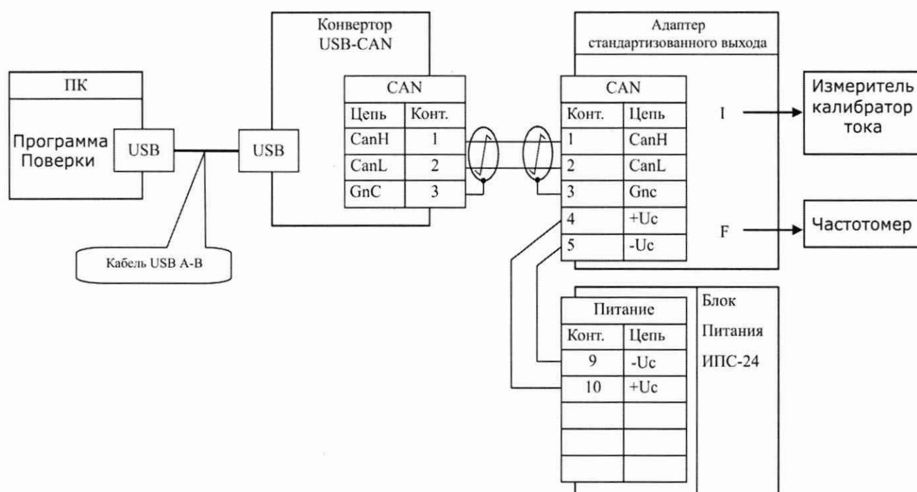
Рисунок Б.6 – Электрическая схема поверки токового и частотного выхода при использовании устройства расширения – адаптера стандартизованных выходов
