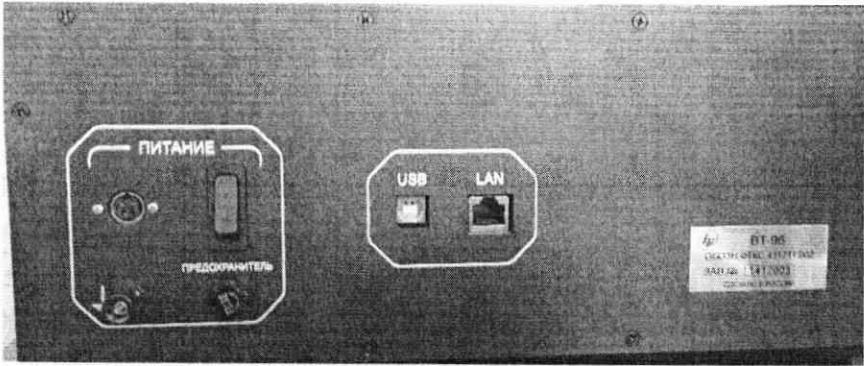
Рисунок 3 – Задняя сторона ВТ-96
