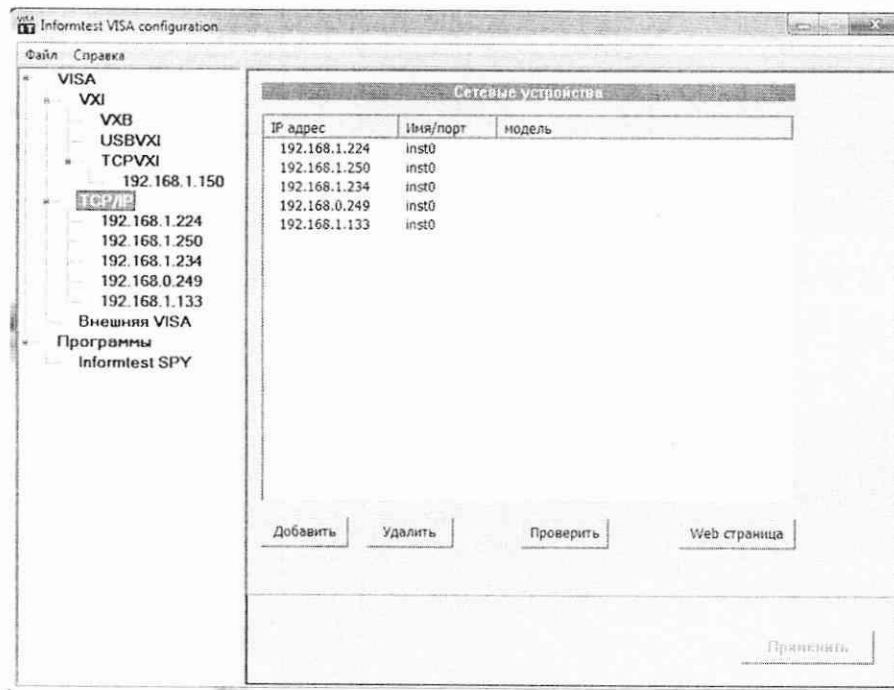
Рисунок 5 – Программная вкладка TCP/IP
