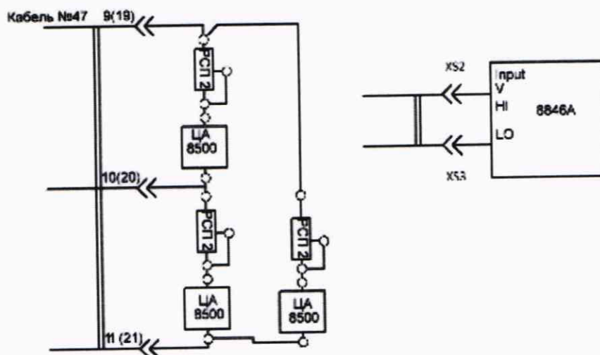
Рисунок 11 – Схема измерений для определения погрешности воспроизведения и измерений среднеквадратического значения напряжения переменного тока между фазами «А» и «В», «В» и «С», «С» и «А»
