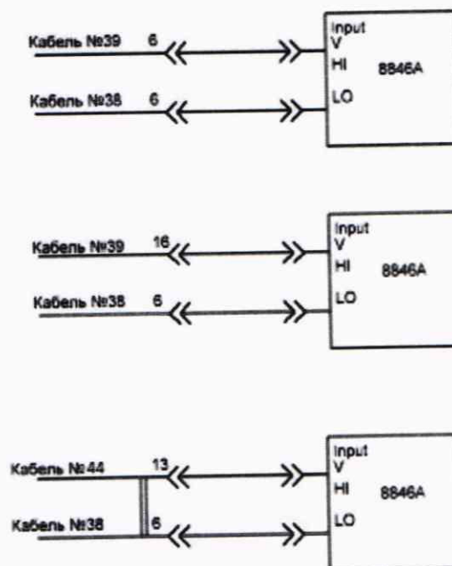
Рисунок 12 – Схемы измерений для определения погрешности воспроизведения дискретных значений напряжения постоянного тока.
