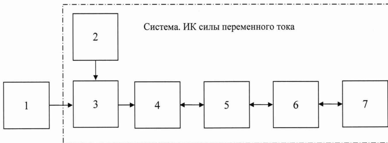
Рисунок Б.5.1 – Функциональная схема поверки ИК напряжения переменного электрического тока
