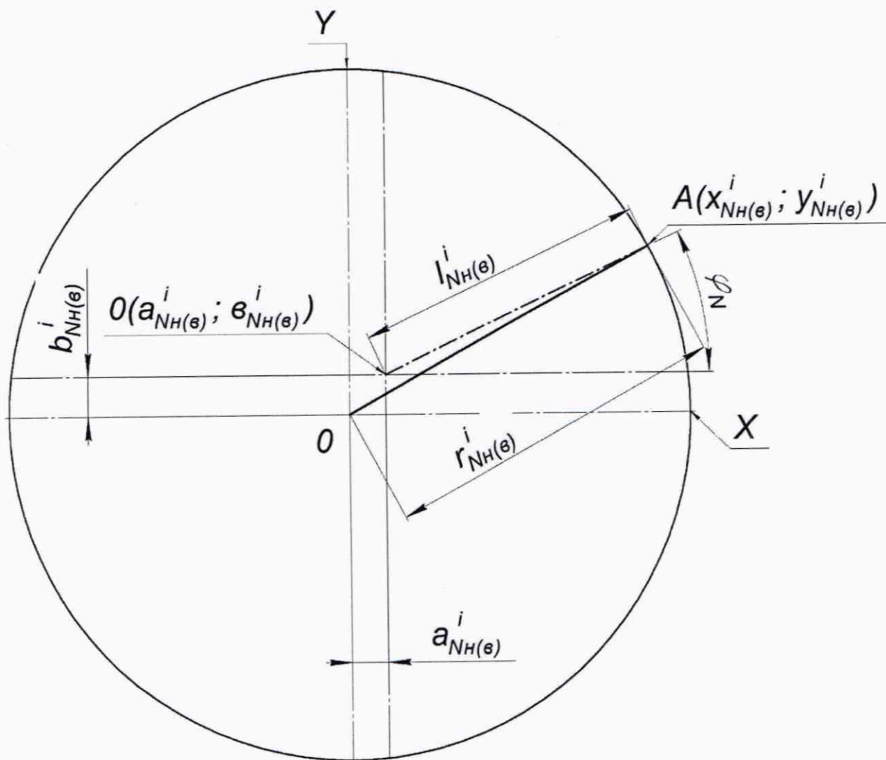
Рисунок Д.1 – Параметры измерений радиуса r_{NH(θ)}^i i -го пояса при j -ом измерении в нижнем (верхнем) сечении
