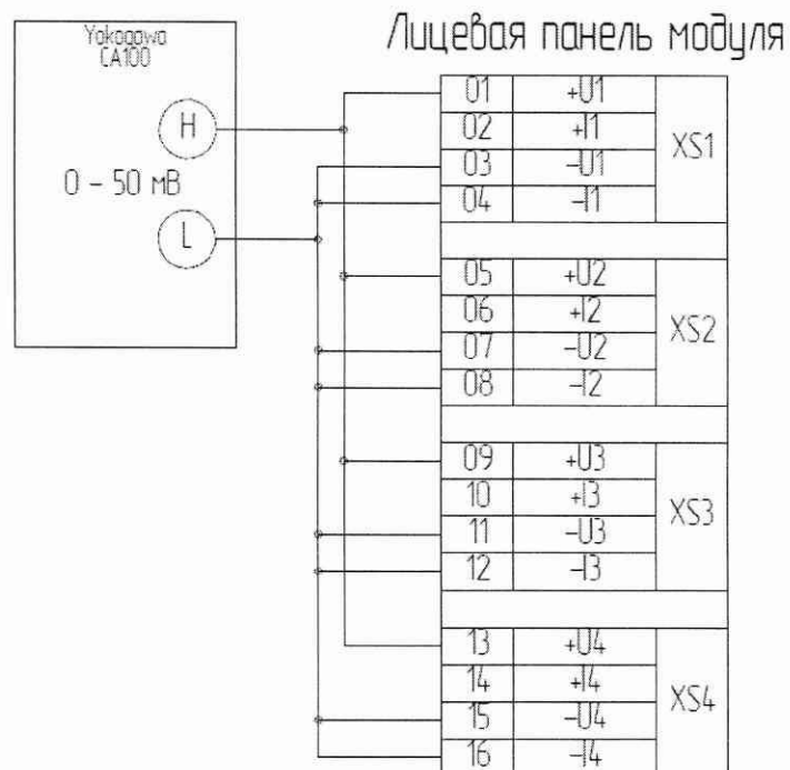
Рисунок А.9 – Пример подключения имитатора (Yokogawa CA100) к модулю AI104 для задания сигналов имитации напряжения постоянного тока (0-50) мВ
