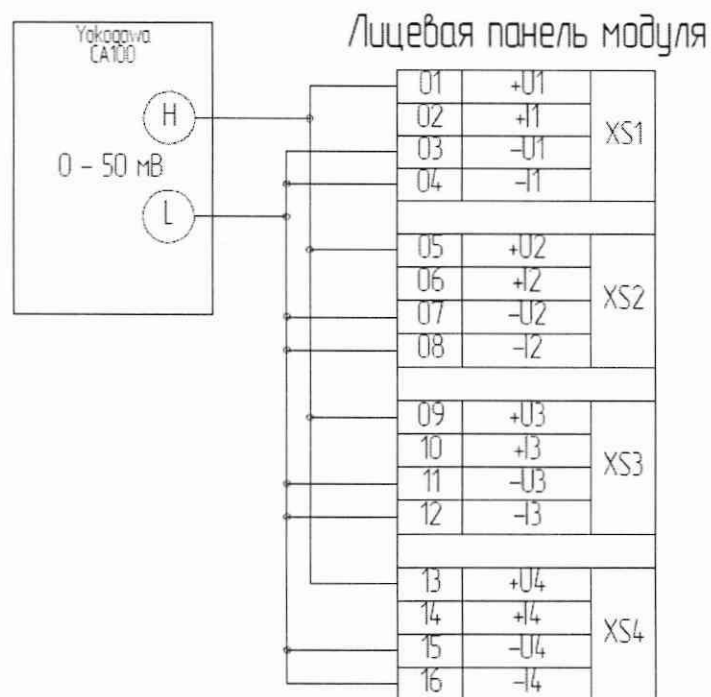
Рисунок А.8 – Пример подключения имитатора (Yokogawa CA100) к модулю AI204 для задания сигналов имитации ЭДС термopар ТХА, ТХК, ТПР (тип В), ТПП (тип S), ТПП (тип R)
