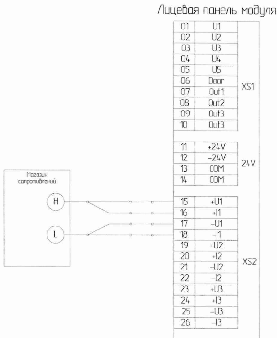
Рисунок А.12 – Пример подключения имитатора (магазин сопротивлений) к модулю SM201 для задания сигналов имитации температуры холодного спая (термопреобразователи сопротивления по ГОСТ6651-2009: Pt-100 \alpha=0,00385 с четырехпроводной схемой подключения)
