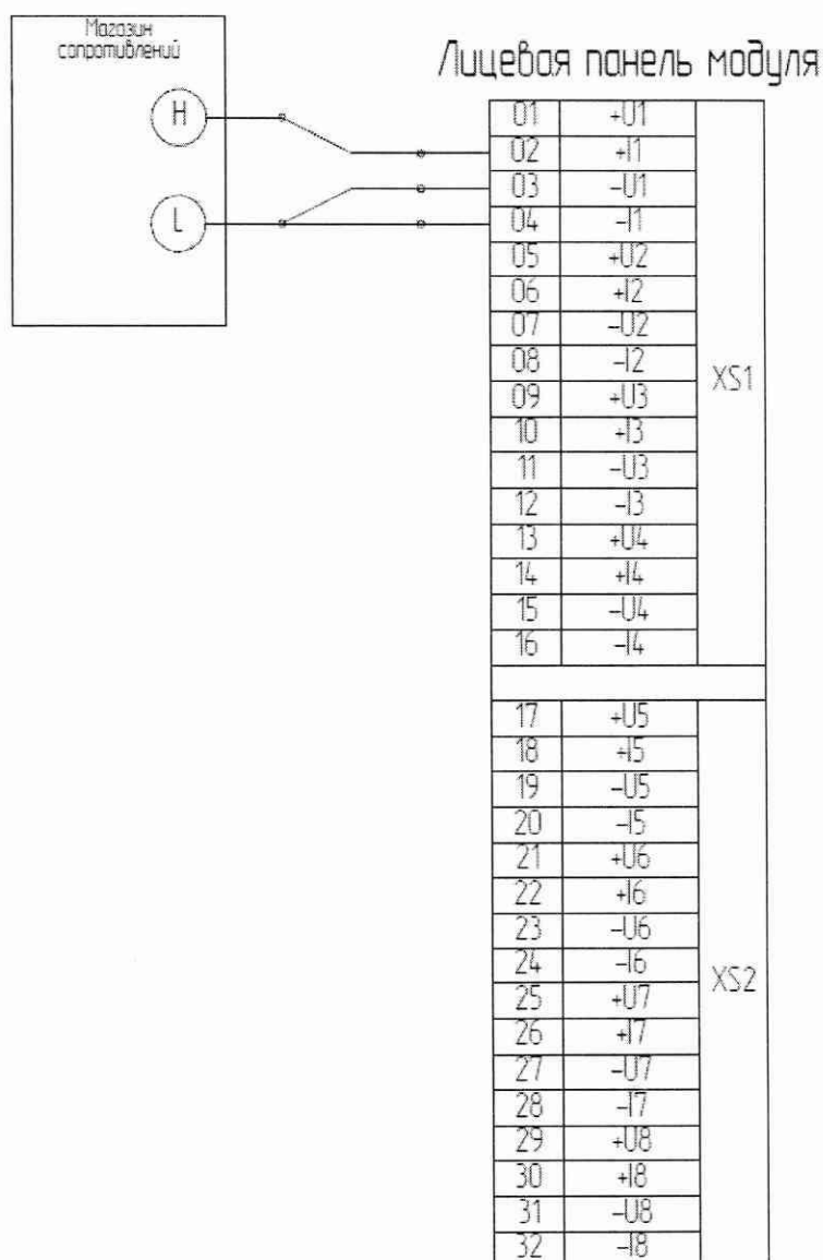
Рисунок А.6 – Пример подключения имитатора (магазин сопротивлений) к модулю AI202 для задания сигналов имитации термопреобразователей ТСМ и ТСП, подключенных по трехпроводной схеме подключения
