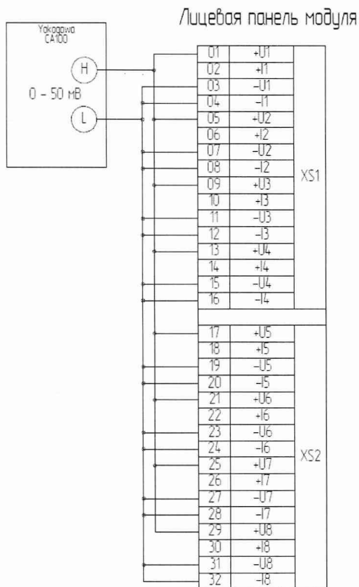
Рисунок А.4 – Пример подключения имитатора (Yokogawa CA100) к модулю AI202 для задания сигналов имитации ЭДС термопар ТХА, ТХК, ТПР (тип В), ТПП (тип S), ТПП (тип R)
