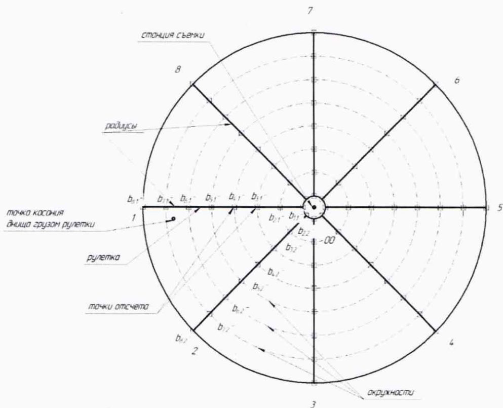
Рисунок А.9 – Координаты отсчета (место установки вехи) неровностей днища
