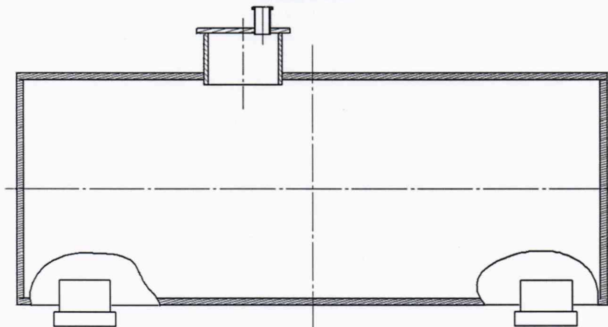
Рисунок А.1 – Общий вид резервуара РГС-4
