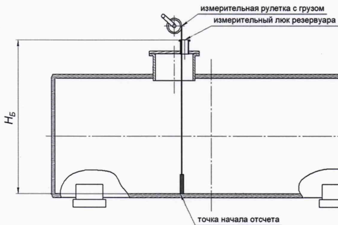
Рисунок А.2 – Схема измерений базовой высоты
