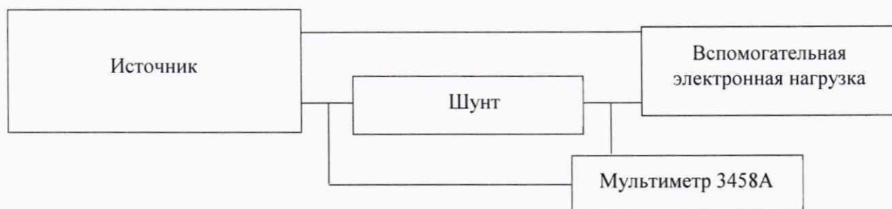
Рисунок 3 – Структурная схема определения абсолютной погрешности воспроизведений/измерений силы постоянного тока
