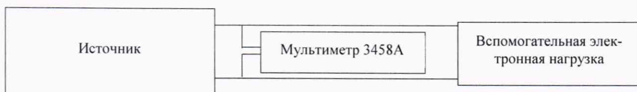
Рисунок 1 – Структурная схема определения абсолютной погрешности воспроизведений/измерений напряжения постоянного тока (от 0 до 1000 В включ.)
