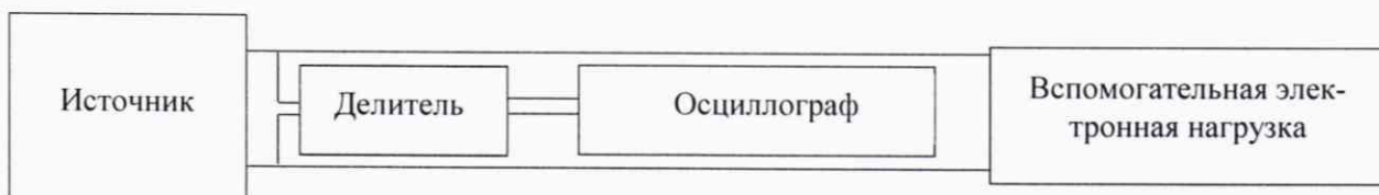
Рисунок 10 - Структурная схема определения уровня пульсаций выходного напряжения постоянного тока в режиме стабилизации напряжения постоянного тока (св. 1000 В)
