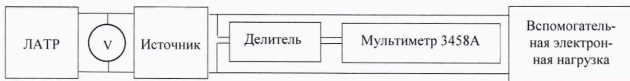
Рисунок 6 - Структурная схема определения неустойчивости выходного напряжения постоянного тока, вызванной изменением напряжения питания (от 0 до 1000 В включ.)
