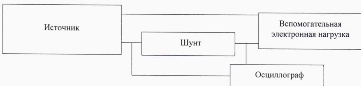
Рисунок 11 - Структурная схема определения уровня пульсаций выходного сигнала силы постоянного тока в режиме стабилизации силы постоянного тока
