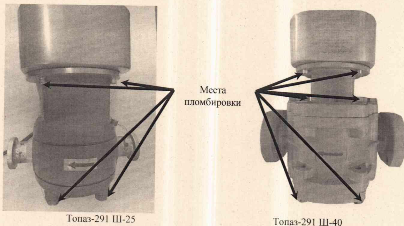
Рисунок 1 - Схемы пломбировки счётчиков
