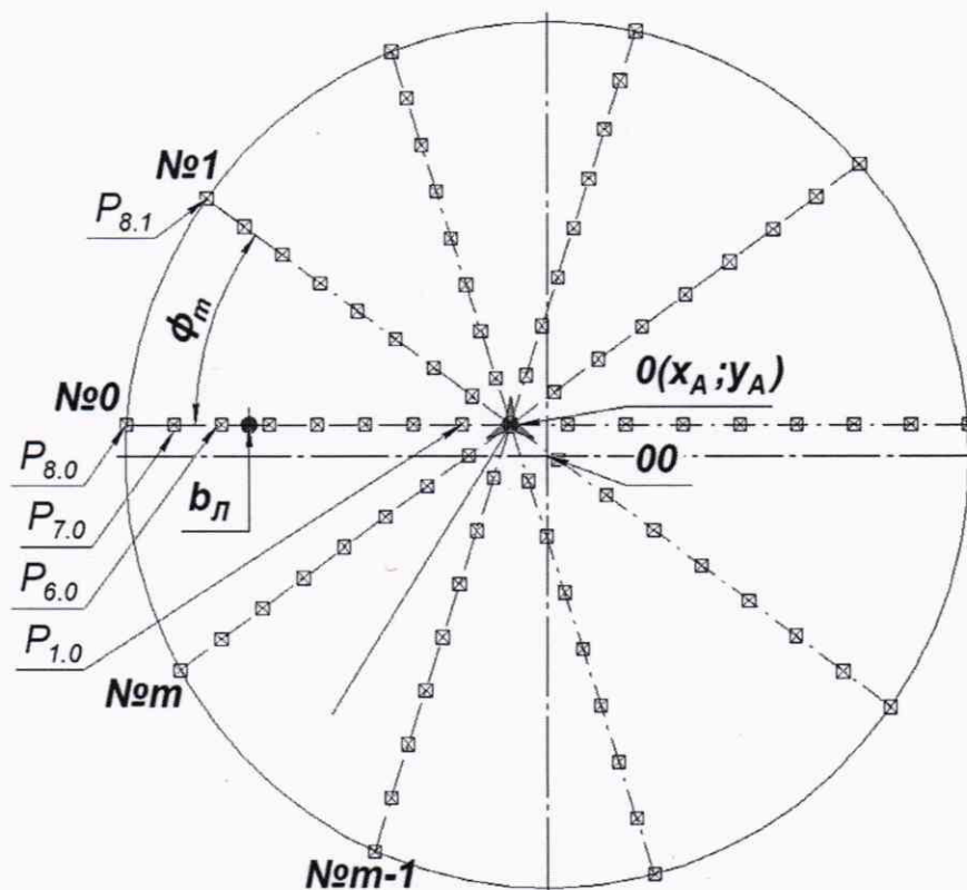
Рисунок А.6.1 – Схема измерений высоты поясов
