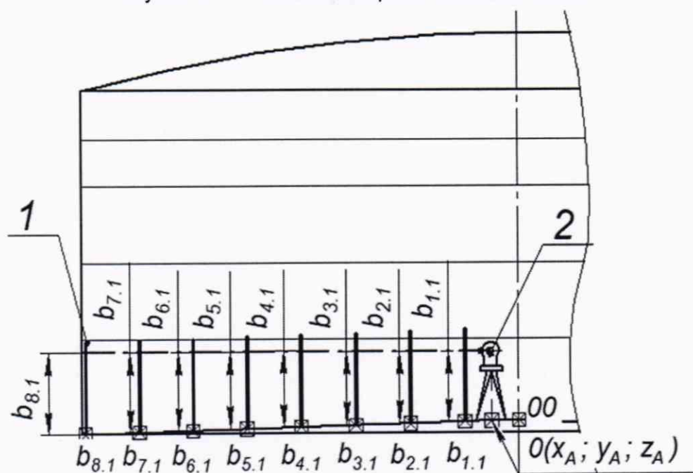
Рисунок А.8 – Рейка нивелирная телескопическая
