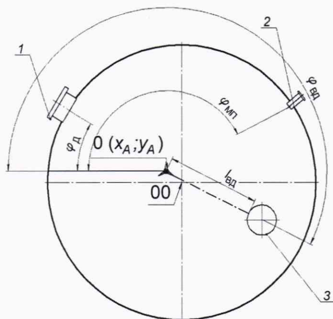
1 – люк-лаз; 2 – приемо-раздаточный патрубок; 3 – внутренняя деталь цилиндрической формы; OO – центр дна резервуара; O(x_A; y_A) – точка установки станции
