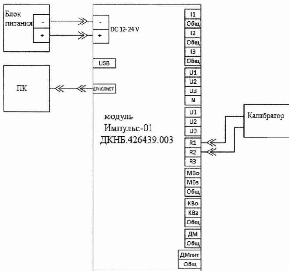
Рисунок 11 – Схема подключения для определения допускаемой основной приведенной погрешности измерений электрического сопротивления постоянному току канала R1-R2
