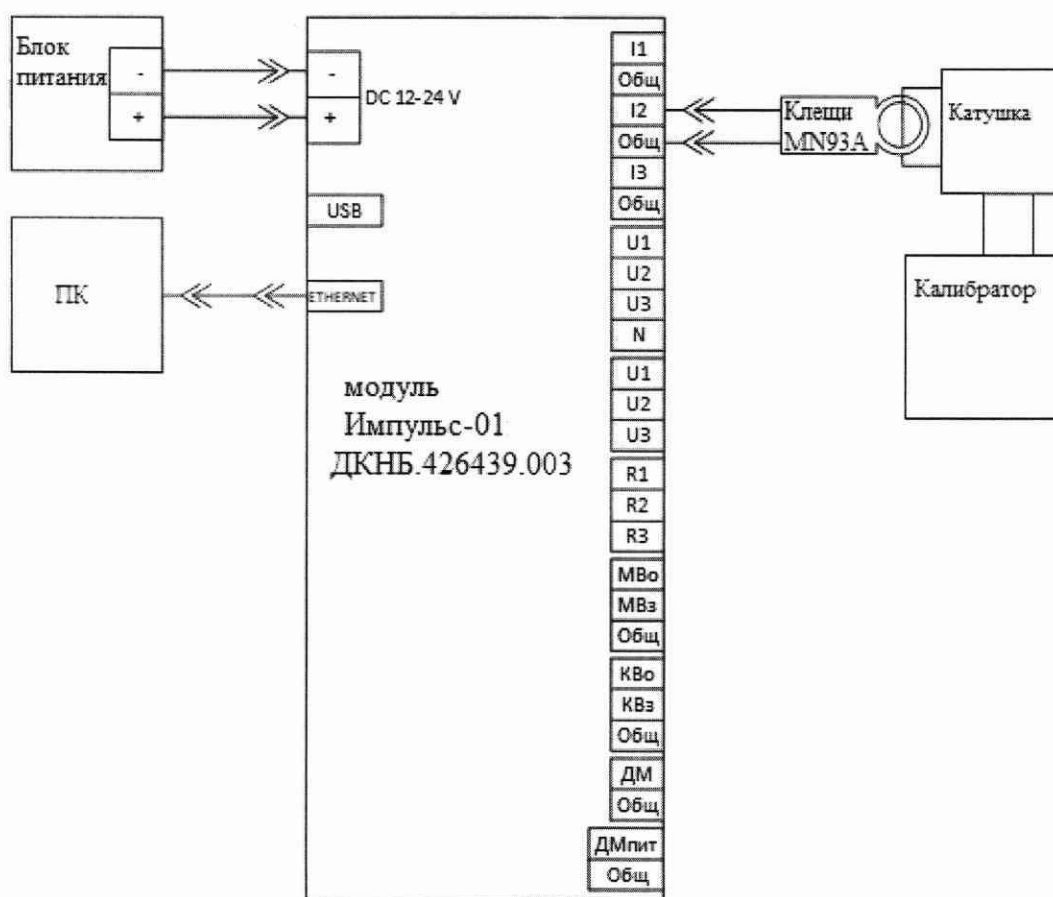
Рисунок 9 – Схема подключения для измерений среднеекватрического значения силы переменного тока канала I_2
