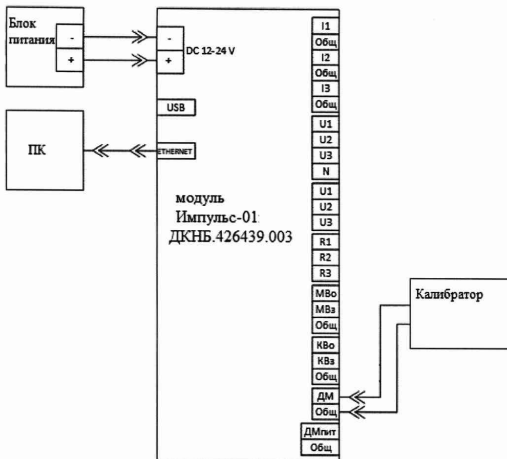
Рисунок 14 – Схема подключения для определения допускаемой относительной погрешности измерений канала датчика крутящего момента
