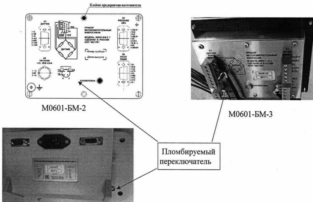
Рисунок 1 — Схема пломбировки от несанкционированного доступа приборов Микросим
