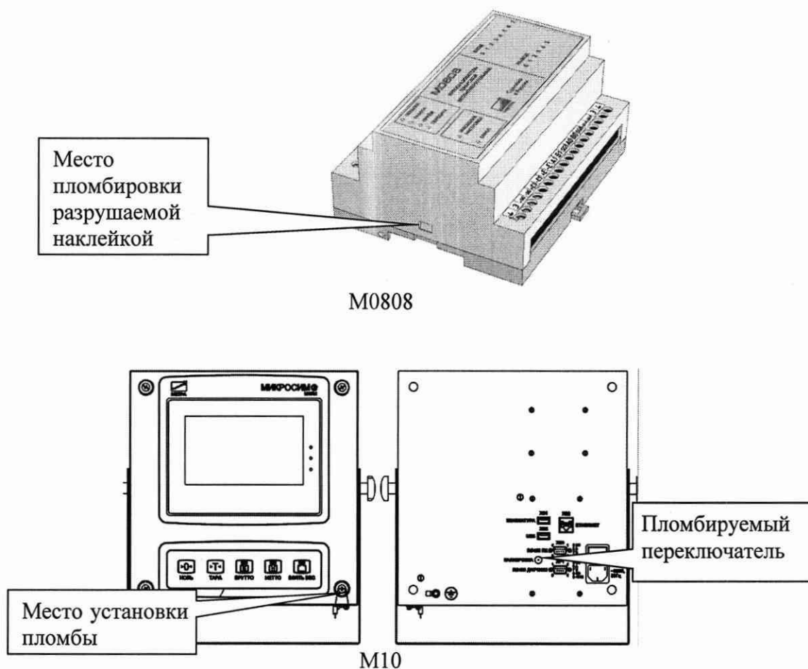
Рисунок 2 — Схема пломбировки от несанкционированного доступа приборов Микросим
