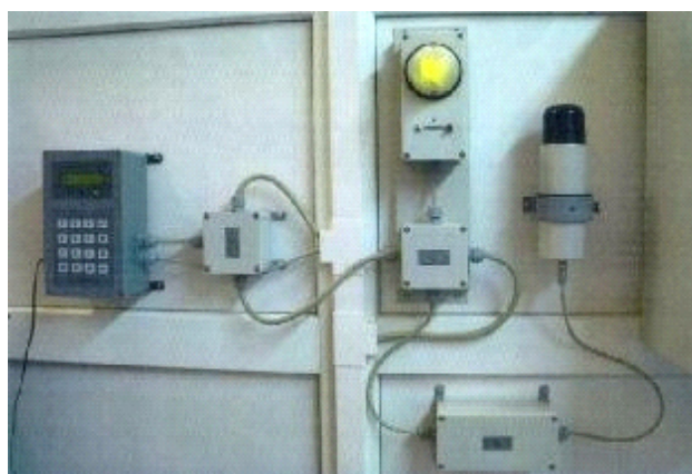
Рис. 4 Система радиационного контроля
